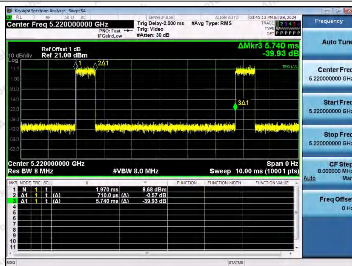
NTNV-11A-Ant1-5220
