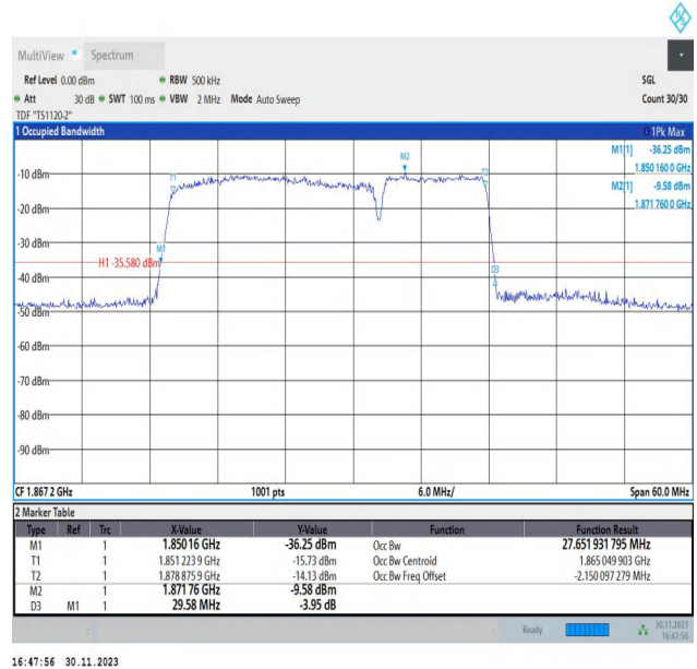
2-2-20MHz-10MHz-16QAM-16QAM-18700-18844-100RB#0-5 0RB#0-PASS
