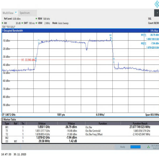
2-2-20MHz-10MHz-QPSK-QPSK-18700-18844-100RB#0-50R B#0-PASS
