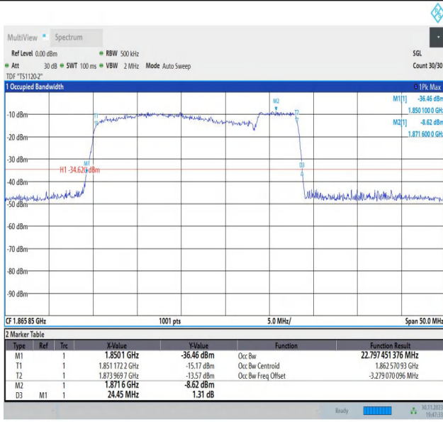
2-2-20MHz-5MHz-16QAM-16QAM-18700-18817-100RB#0-25 RB#0-PASS
