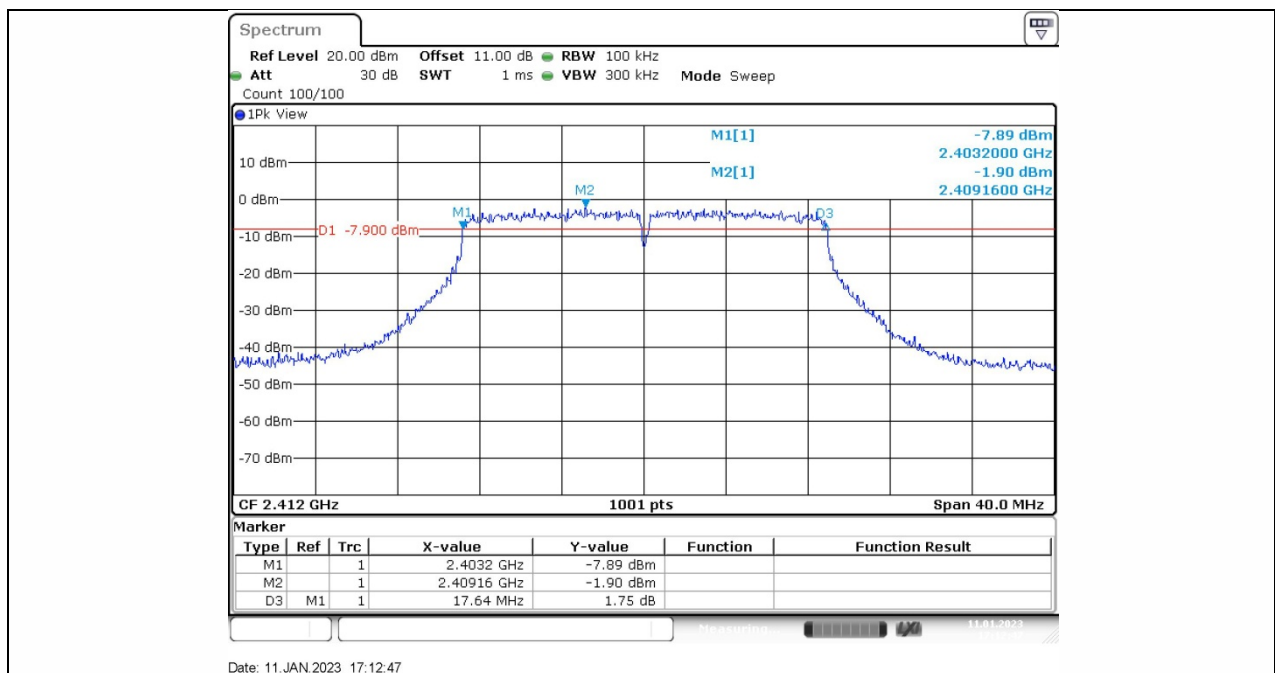
11N20SISO_Ant1_2437
