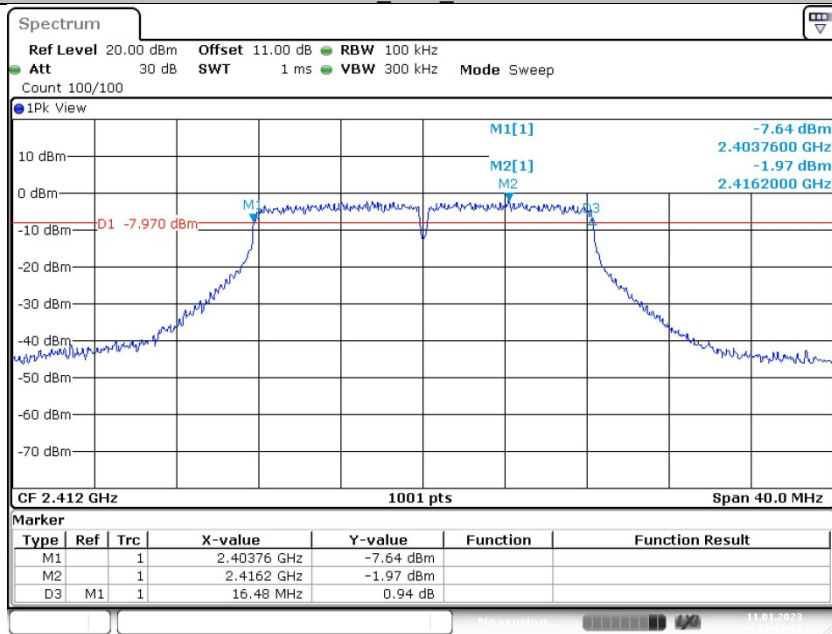
11G_Ant1_2412
