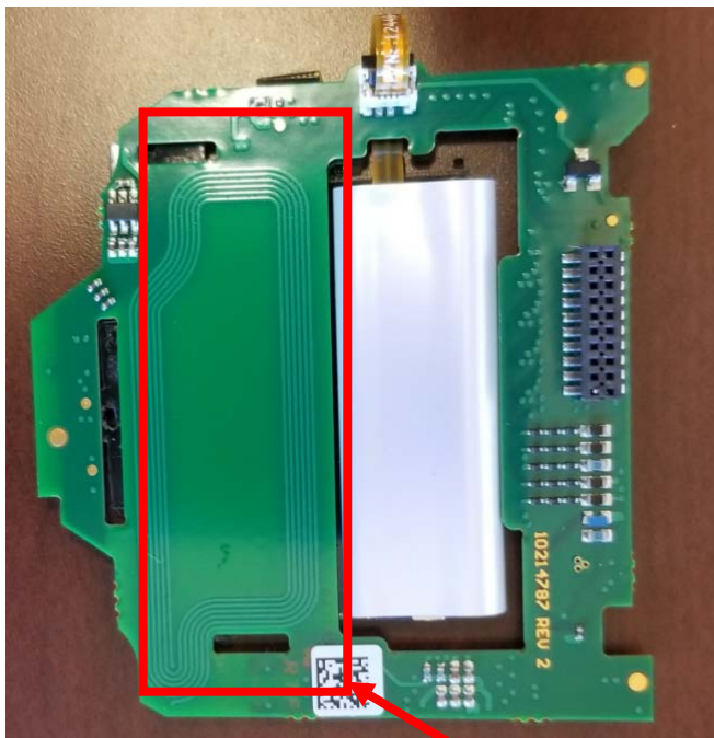
RFID Antenna
