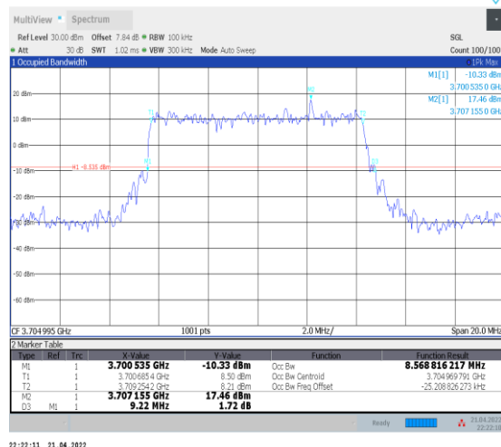
1-N77-3700-3980--30-10-L-2-DFT-PI2BPSK-Outter_Full -24@0-Ant0-8.569-9.220-≤10-PASS
