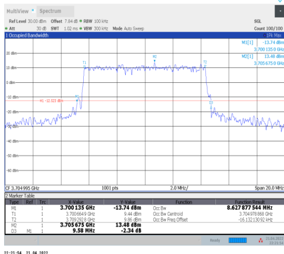
1-N77-3700-3980--30-10-L-1-DFT-QPSK-Outter_Full -24@0-Ant0-8.628-9.580-≤10-PASS
