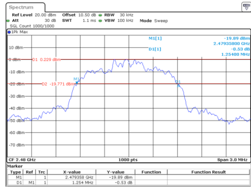
\pi/4 -DQPSK_High 1.254 MHz
