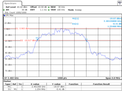
\pi/4 -DQPSK_Low 1.254 MHz
