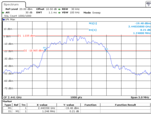
\pi/4 -DQPSK_Middle 1.248 MHz
