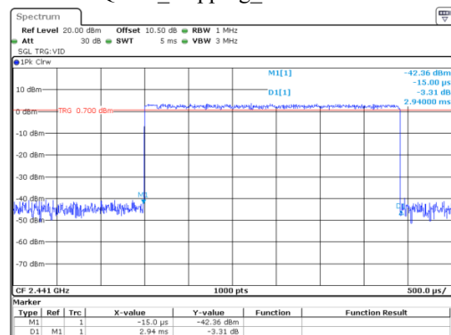
\pi/4 -DQPSK_Hopping_2DH5 2.940ms
