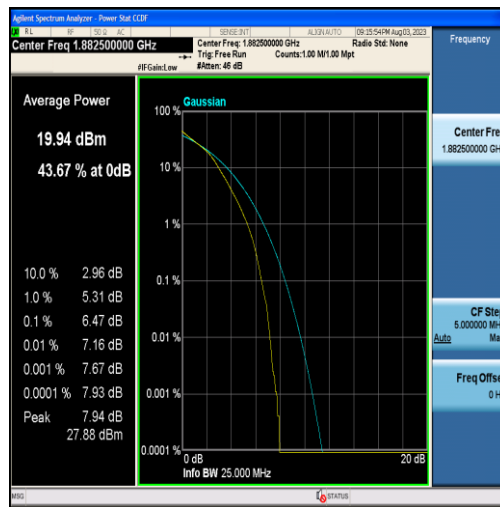
Band25-10MHz-16QAM-26365-50RB#0
