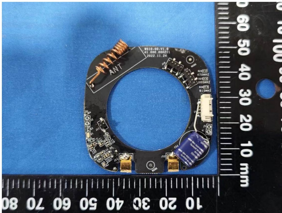
Lora ANT
