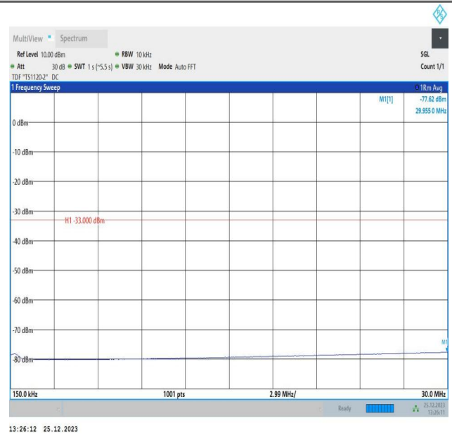
66-66-10MHz-10MHz-QPSK-QPSK-132373-132472-1RB#49- ORB#0-0.15~30MHz-PASS
