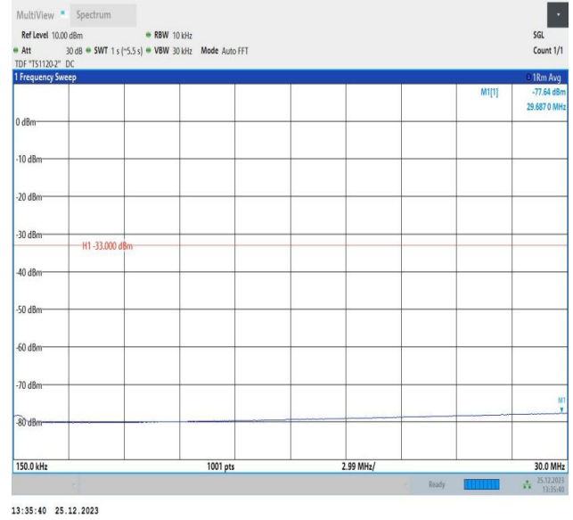
66-66-10MHz-10MHz-QPSK-QPSK-132523-132622-1RB#0-1RB#49-0.15~30MHz-PASS
