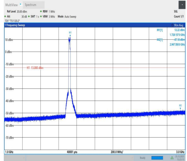
66-66-10MHz-10MHz-QPSK-QPSK-132022-132121-50RB#0- 50RB#0-1000~3000MHz-PASS
