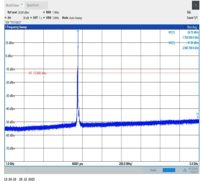
66-66-10MHz-10MHz-QPSK-QPSK-132373-132472-1RB#49- ORB#0-1000~3000MHz-PASS
