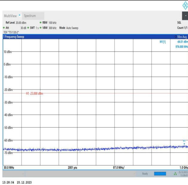
66-66-10MHz-10MHz-QPSK-QPSK-132373-132472-1RB#0-1RB#49-30~1000MHz-PASS
