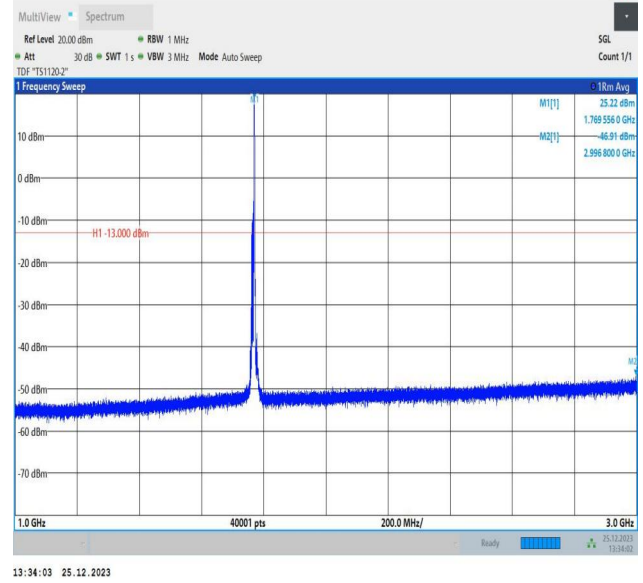
66-66-10MHz-10MHz-QPSK-QPSK-132523-132622-1RB#49- ORB#0-1000~3000MHz-PASS
