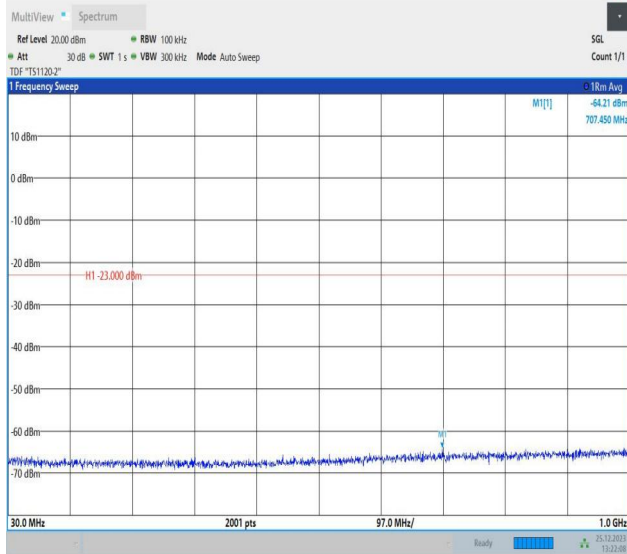
66-66-10MHz-10MHz-QPSK-QPSK-132022-132121-50RB#0 -50RB#0-30~1000MHz-PASS
