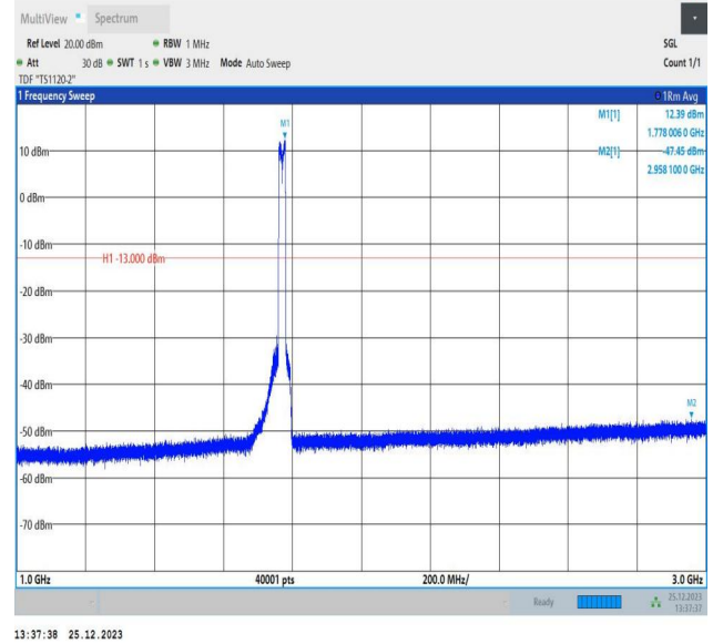
66-66-10MHz-10MHz-QPSK-QPSK-132523-132622-50RB#0-50RB#0-1000~3000MHz-PASS
