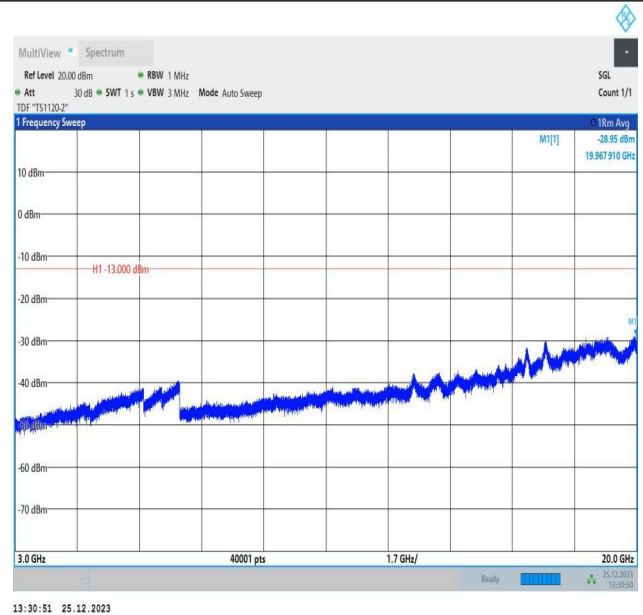
66-66-10MHz-10MHz-16QAM-16QAM-132373-132472-50RB #0-50RB#0-3000~20000MHz-PASS
