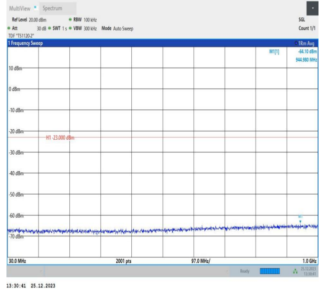
66-66-10MHz-10MHz-16QAM-16QAM-132373-132472-50RB #0-50RB#0-30~1000MHz-PASS
