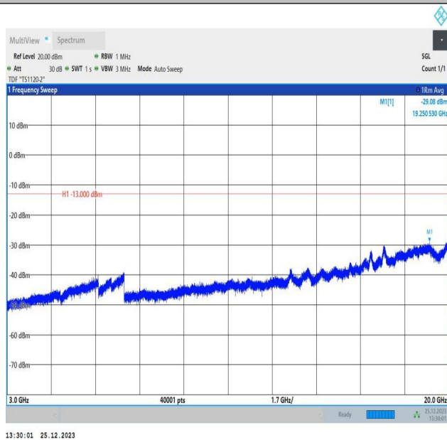
66-66-10MHz-10MHz-QPSK-QPSK-132373-132472-50RB#0 -50RB#0-3000~20000MHz-PASS
