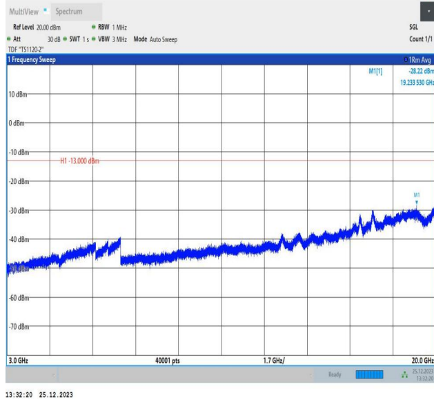
66-66-10MHz-10MHz-QPSK-QPSK-132523-132622-1RB#0-ORB#0-3000~20000MHz-PASS
