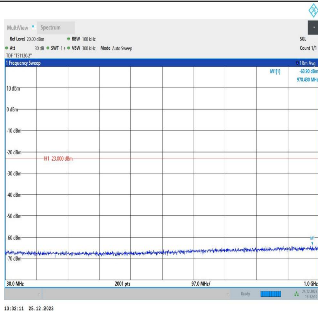
66-66-10MHz-10MHz-QPSK-QPSK-132523-132622-1RB#0-0RB#0-30~1000MHz-PASS
