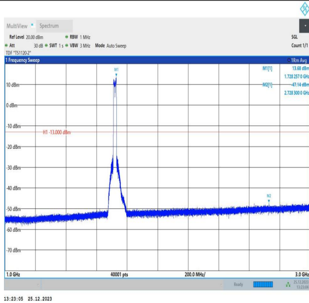
66-66-10MHz-10MHz-16QAM-16QAM-132022-132121-50RB #0-50RB#0-1000~3000MHz-PASS
