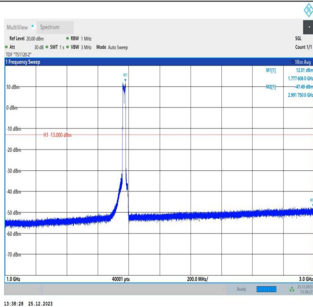
66-66-10MHz-10MHz-16QAM-16QAM-132523-132622-50RB #0-50RB#0-1000~3000MHz-PASS
