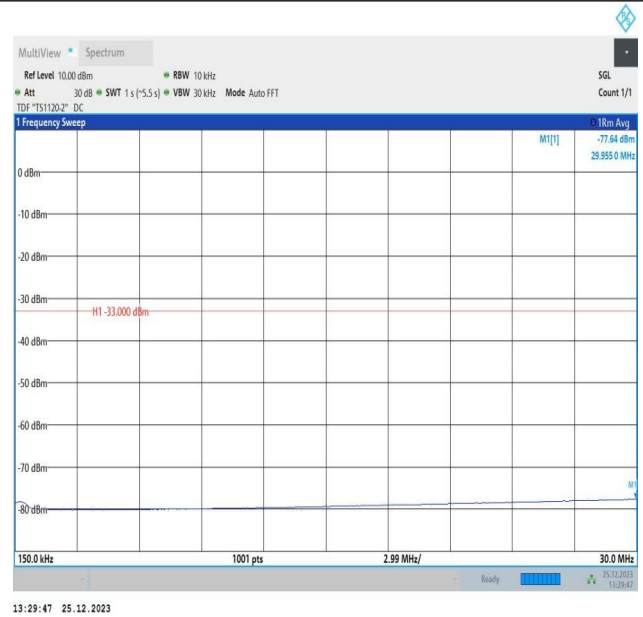
66-66-10MHz-10MHz-QPSK-QPSK-132373-132472-50RB#0- 50RB#0-0.15~30MHz-PASS
