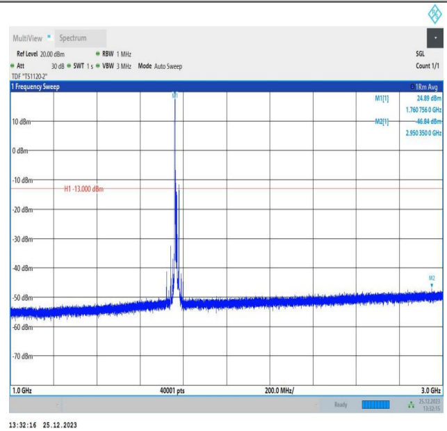
66-66-10MHz-10MHz-QPSK-QPSK-132523-132622-1RB#0-0RB#0-1000~3000MHz-PASS
