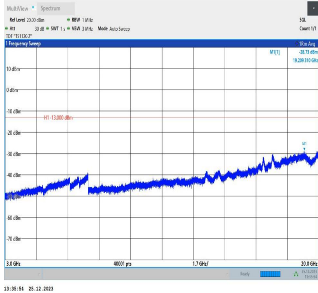
66-66-10MHz-10MHz-QPSK-QPSK-132523-132622-1RB#0-1RB#49-3000~20000MHz-PASS
