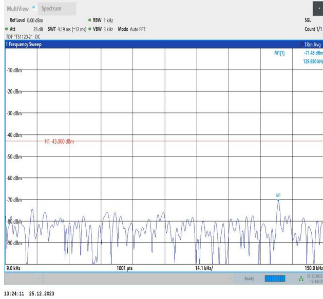
66-66-10MHz-10MHz-QPSK-QPSK-132373-132472-1RB#0-0RB#0-0.009~0.15MHz-PASS
