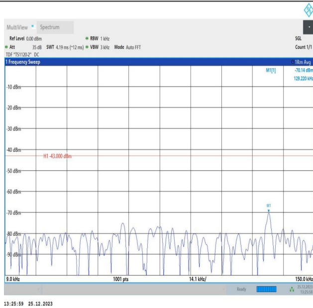
66-66-10MHz-10MHz-QPSK-QPSK-132373-132472-1RB#49 -ORB#0-0.009~0.15MHz-PASS
