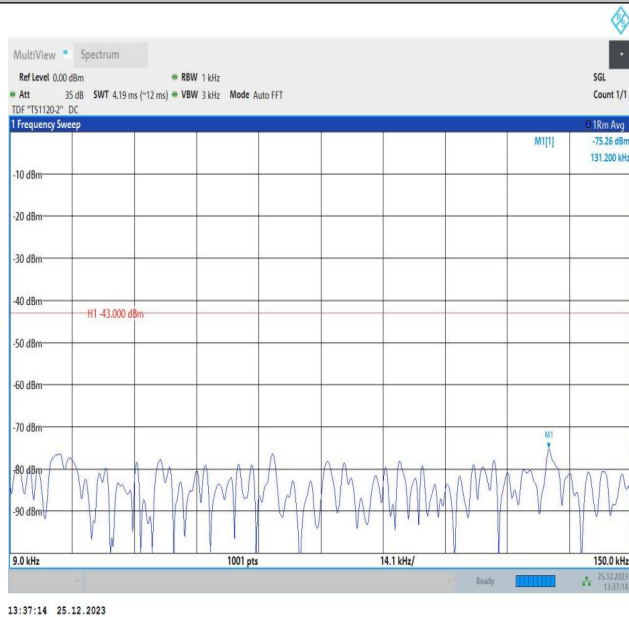
66-66-10MHz-10MHz-QPSK-QPSK-132523-132622-50RB#0 -50RB#0-0.009~0.15MHz-PASS
