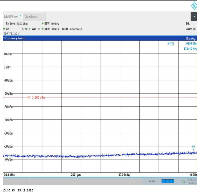
66-66-10MHz-10MHz-QPSK-QPSK-132523-132622-1RB#0-1RB#49-30~1000MHz-PASS
