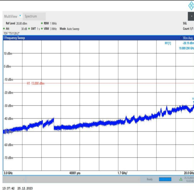
66-66-10MHz-10MHz-QPSK-QPSK-132523-132622-50RB#0-50RB#0-3000~20000MHz-PASS
