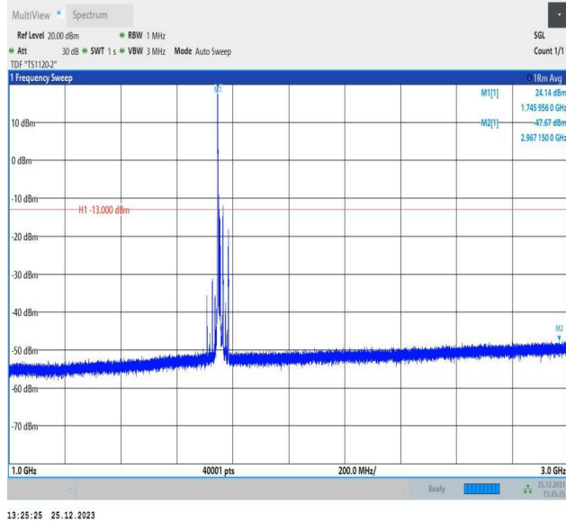
66-66-10MHz-10MHz-16QAM-16QAM-132373-132472-1RB# 0-ORB#0-1000~3000MHz-PASS
