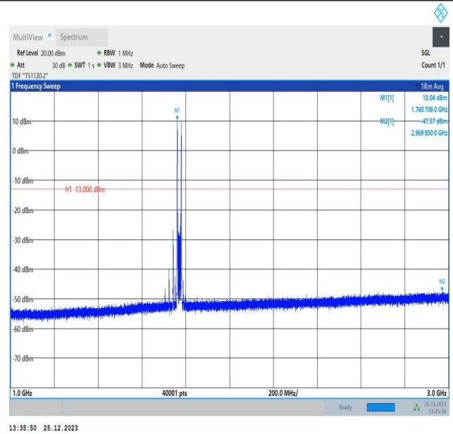
66-66-10MHz-10MHz-QPSK-QPSK-132523-132622-1RB#0-1RB#49-1000~3000MHz-PASS
