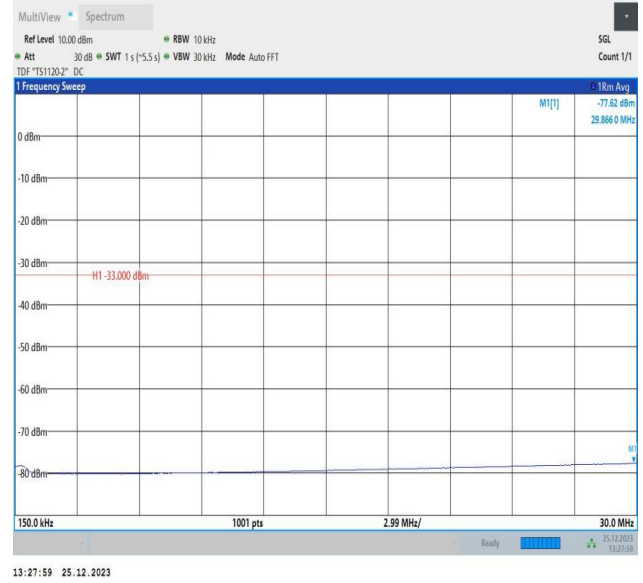
66-66-10MHz-10MHz-QPSK-QPSK-132373-132472-1RB#0-1RB#49-0.15~30MHz-PASS
