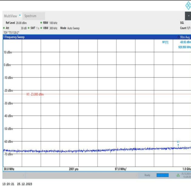
66-66-10MHz-10MHz-QPSK-QPSK-132022-132121-1RB#0-1RB#49-30~1000MHz-PASS
