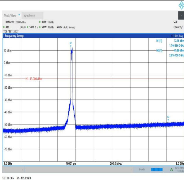
66-66-10MHz-10MHz-16QAM-16QAM-132373-132472-50RB #0-50RB#0-1000~3000MHz-PASS
