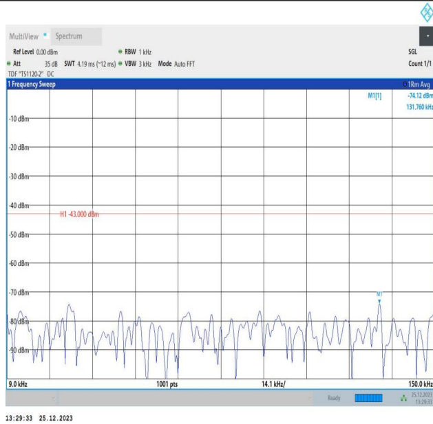
66-66-10MHz-10MHz-QPSK-QPSK-132373-132472-50RB#0 -50RB#0-0.009~0.15MHz-PASS
