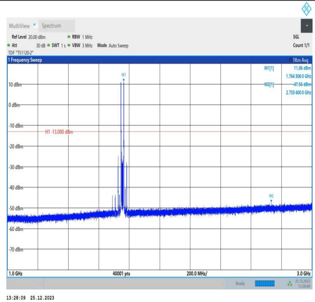
66-66-10MHz-10MHz-QPSK-QPSK-132373-132472-1RB#0-1RB#49-1000~3000MHz-PASS
