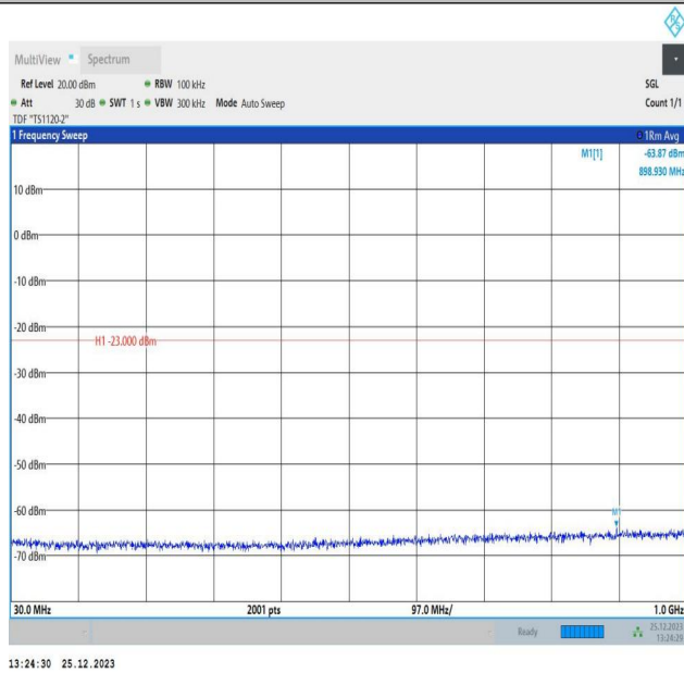
66-66-10MHz-10MHz-QPSK-QPSK-132373-132472-1RB#0-0RB#0-30~1000MHz-PASS
