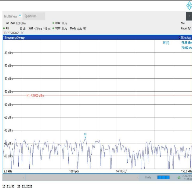
66-66-10MHz-10MHz-QPSK-QPSK-132022-132121-50RB#0 -50RB#0-0.009~0.15MHz-PASS
