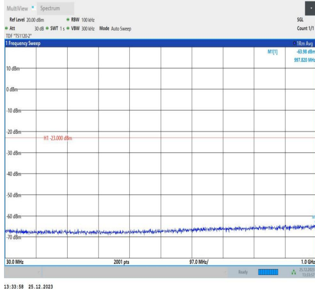
66-66-10MHz-10MHz-QPSK-QPSK-132523-132622-1RB#49 -ORB#0-30~1000MHz-PASS
