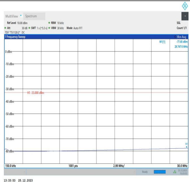
66-66-10MHz-10MHz-QPSK-QPSK-132523-132622-1RB#49- ORB#0-0.15~30MHz-PASS
