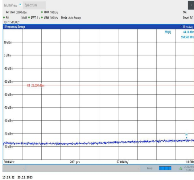
66-66-10MHz-10MHz-QPSK-QPSK-132373-132472-50RB#0 -50RB#0-30~1000MHz-PASS
