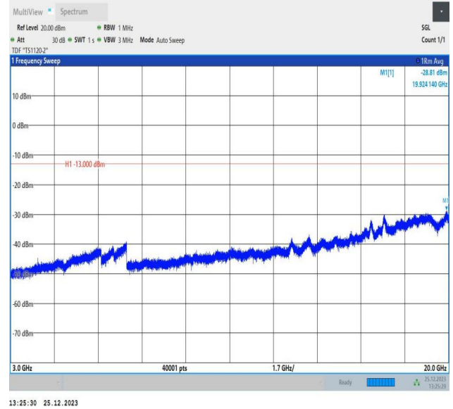
66-66-10MHz-10MHz-16QAM-16QAM-132373-132472-1RB# 0-ORB#0-3000~20000MHz-PASS
