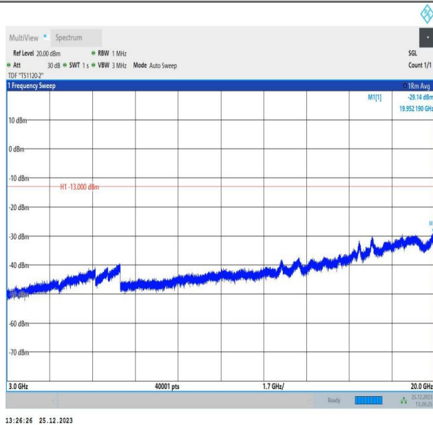
66-66-10MHz-10MHz-QPSK-QPSK-132373-132472-1RB#49 -ORB#0-3000~20000MHz-PASS
