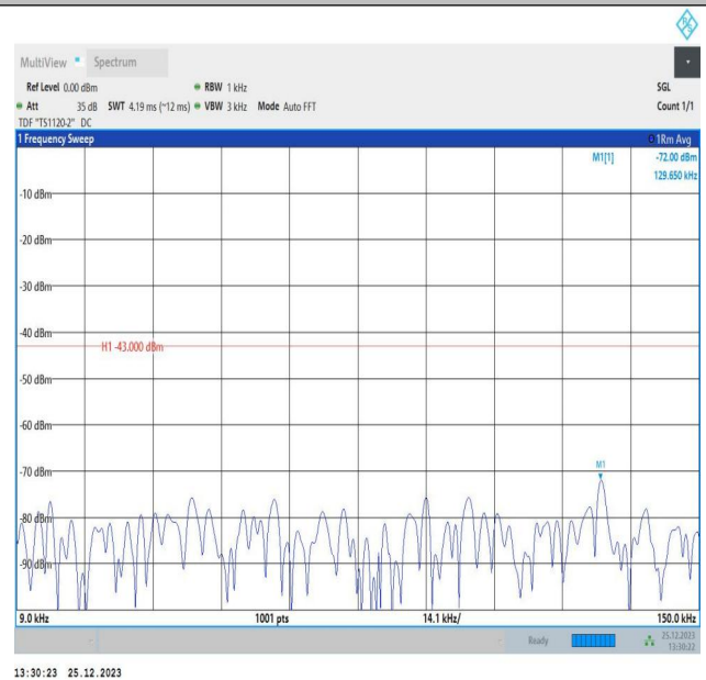
66-66-10MHz-10MHz-16QAM-16QAM-132373-132472-50RB #0-50RB#0-0.009~0.15MHz-PASS
