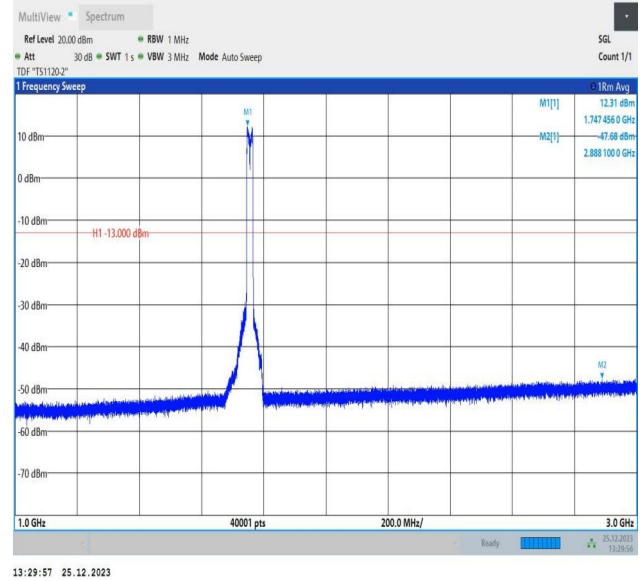
66-66-10MHz-10MHz-QPSK-QPSK-132373-132472-50RB#0- 50RB#0-1000~3000MHz-PASS
