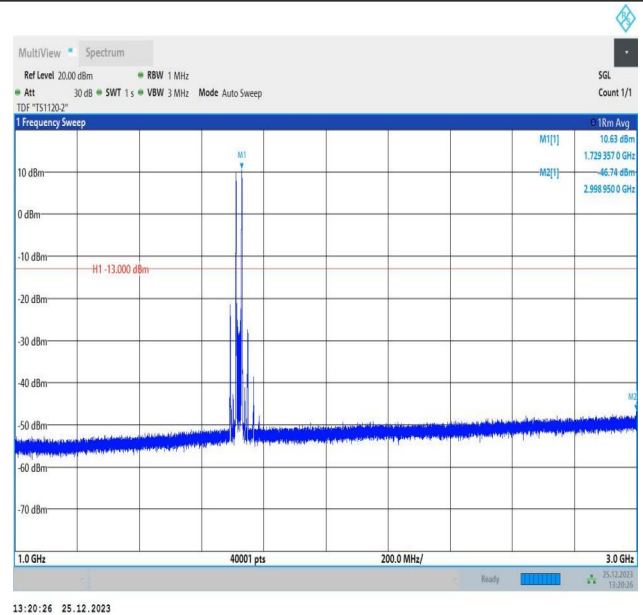
66-66-10MHz-10MHz-QPSK-QPSK-132022-132121-1RB#0-1RB#49-1000~3000MHz-PASS
