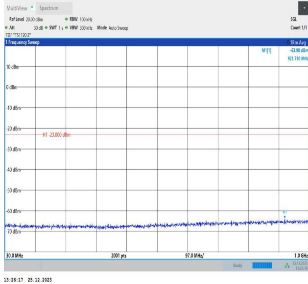
66-66-10MHz-10MHz-QPSK-QPSK-132373-132472-1RB#49 -ORB#0-30~1000MHz-PASS
