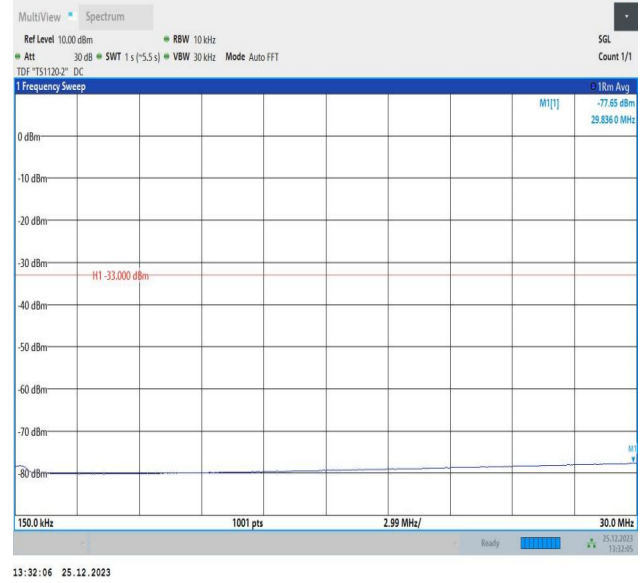
66-66-10MHz-10MHz-QPSK-QPSK-132523-132622-1RB#0-0RB#0-0.15~30MHz-PASS
