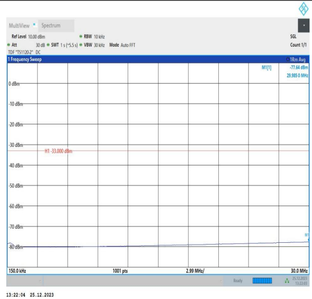
66-66-10MHz-10MHz-QPSK-QPSK-132022-132121-50RB#0- 50RB#0-0.15~30MHz-PASS
