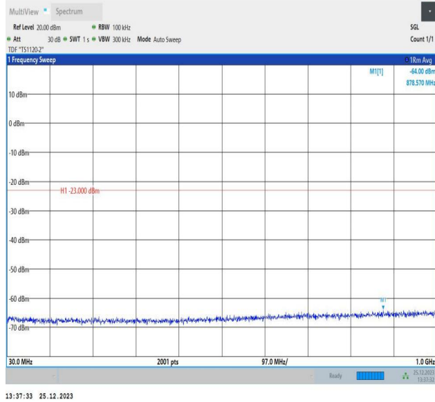
66-66-10MHz-10MHz-QPSK-QPSK-132523-132622-50RB#0-50RB#0-30~1000MHz-PASS
