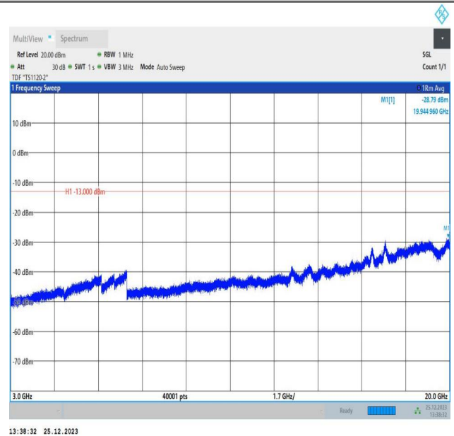
66-66-10MHz-10MHz-16QAM-16QAM-132523-132622-50RB #0-50RB#0-3000~20000MHz-PASS
