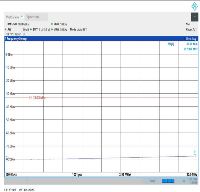
66-66-10MHz-10MHz-QPSK-QPSK-132523-132622-50RB#0- 50RB#0-0.15~30MHz-PASS
