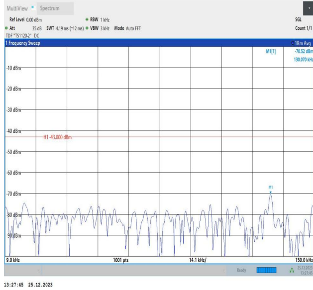
66-66-10MHz-10MHz-QPSK-QPSK-132373-132472-1RB#0-1RB#49-0.009~0.15MHz-PASS
