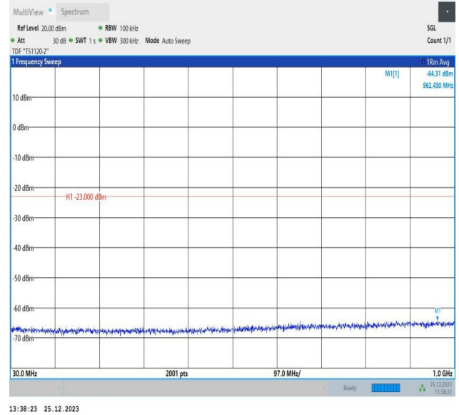
66-66-10MHz-10MHz-16QAM-16QAM-132523-132622-50RB #0-50RB#0-30~1000MHz-PASS
