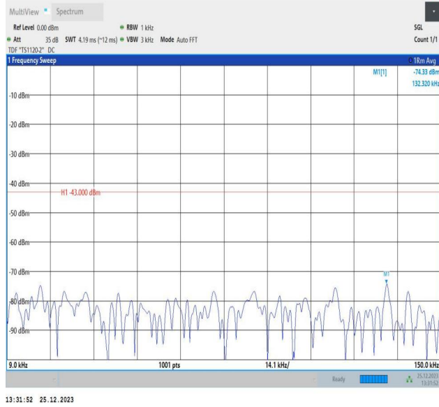
66-66-10MHz-10MHz-QPSK-QPSK-132523-132622-1RB#0-0RB#0-0.009~0.15MHz-PASS
