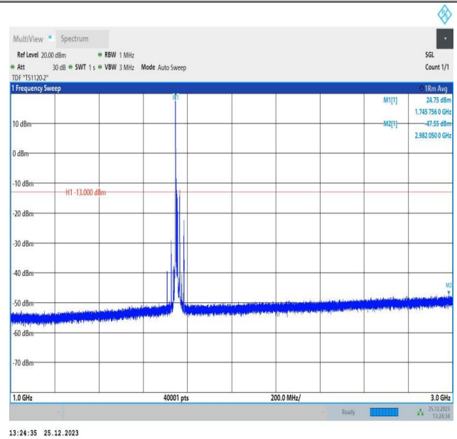
66-66-10MHz-10MHz-QPSK-QPSK-132373-132472-1RB#0-0RB#0-1000~3000MHz-PASS
