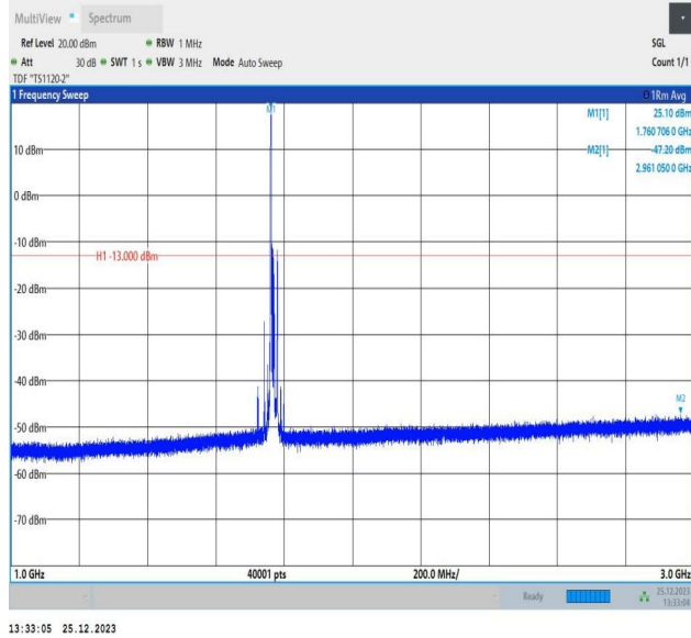
66-66-10MHz-10MHz-16QAM-16QAM-132523-132622-1RB# 0-ORB#0-1000~3000MHz-PASS
