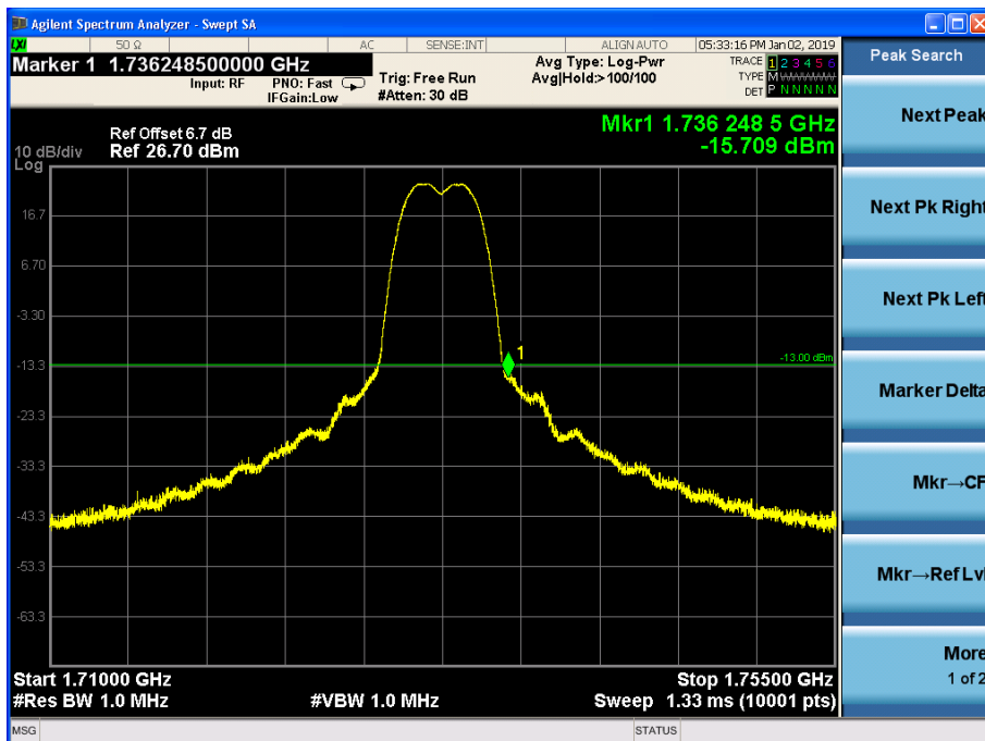
Channel 1412, 1710MHz~1755MHz
