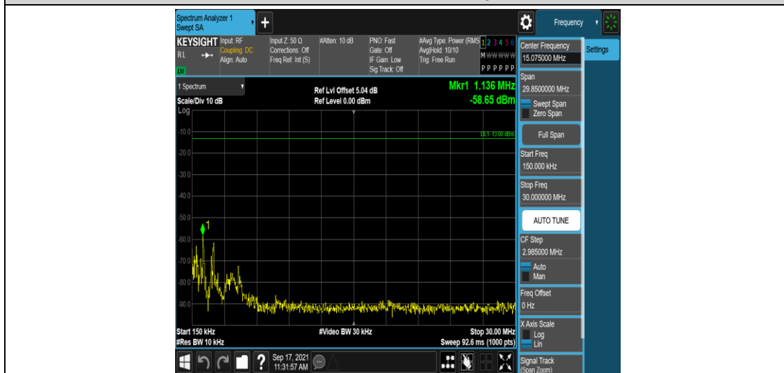
Band12-5MHz-QPSK-23095-1RB#0-Range2:0.15~30MHz
