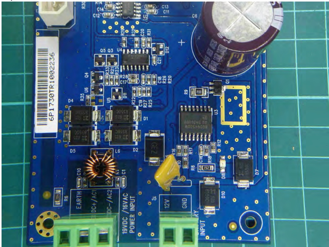
(272) EUT Photo
