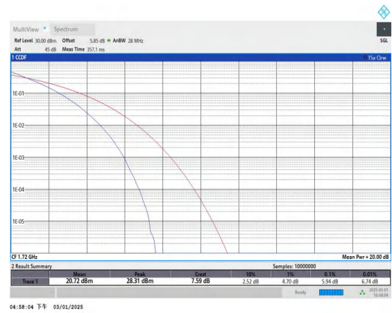
Band4-20MHz-QPSK-20050-100RB#0-PASS
