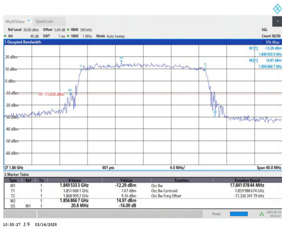
Band2-20MHz-QPSK-18700-100RB#0-PASS
