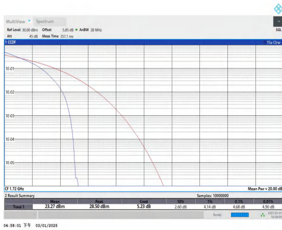
Band4-20MHz-QPSK-20050-1RB#0-PASS
