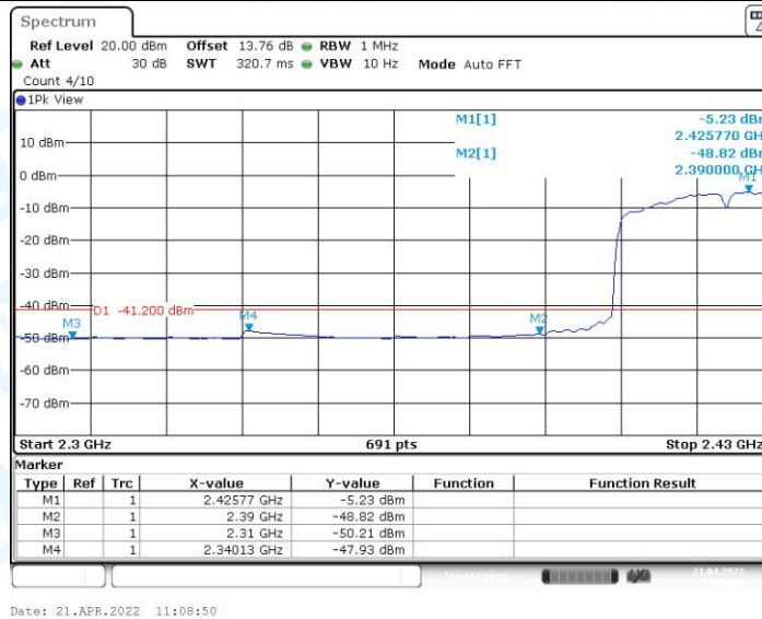
11N40SISO_Ant1_Low_2422_AV
