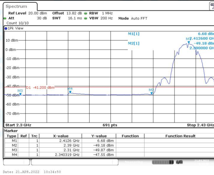
11B_Ant1_Low_2412_AV
