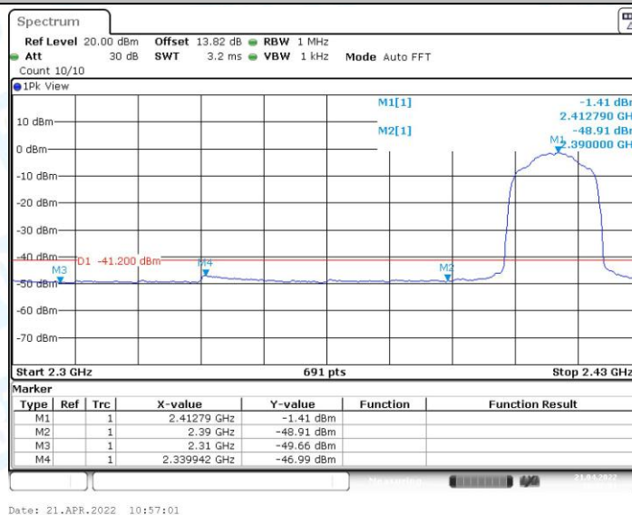
11N20SISO_Ant1_Low_2412_AV
