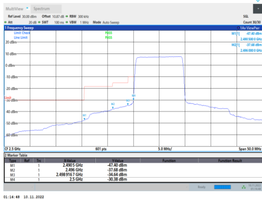
Band7-10MHz-QPSK-20800-50RB#0
