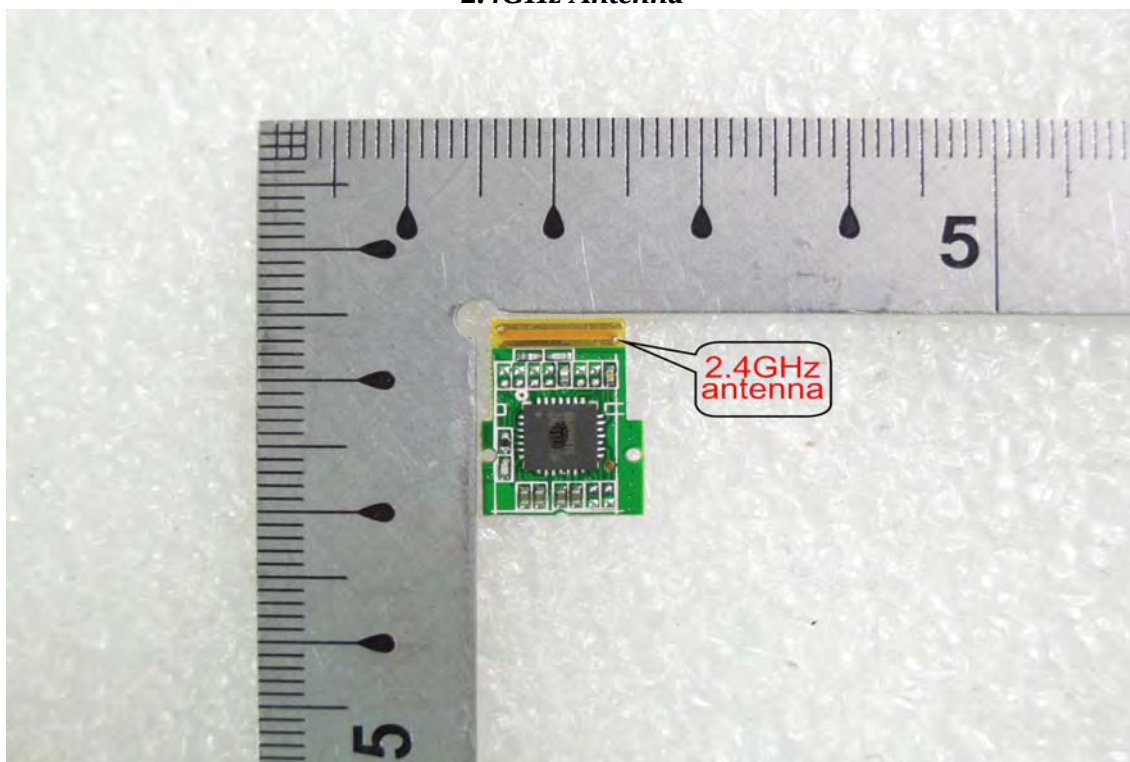
2.4GHz Antenna
