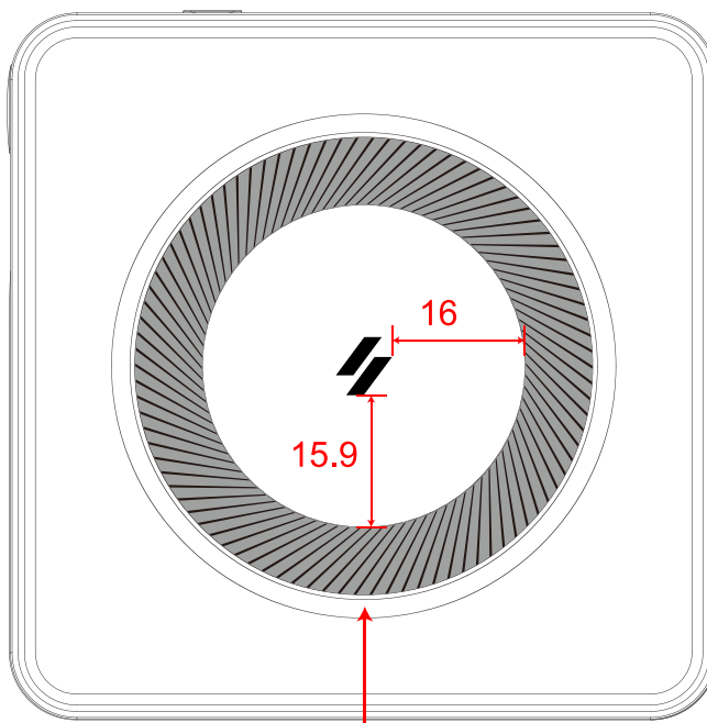
後視圖
