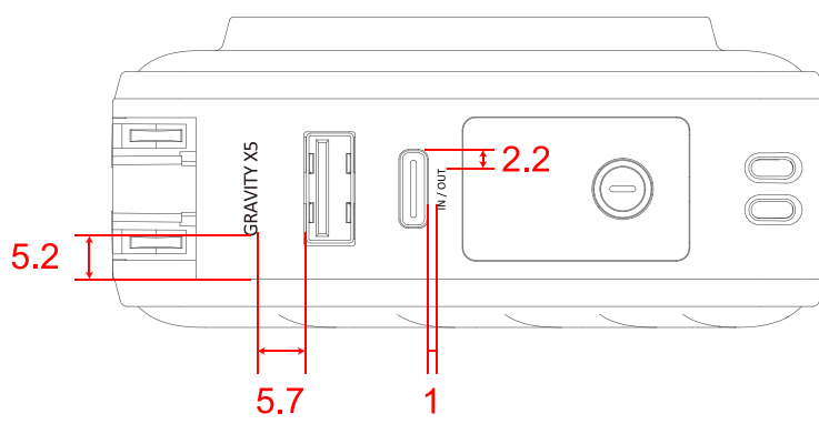
上視圖
