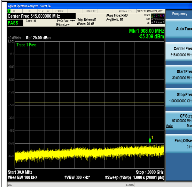
NTNV-n77(3700-3980)-PC2-30-100-L-CP-QPSK- Edge_1RB_Left-30-1000-PASS
