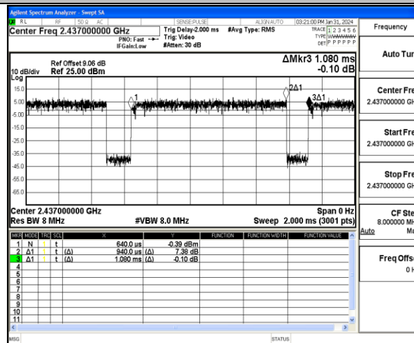
NTNV-11N40MIMO-Ant1-2437
