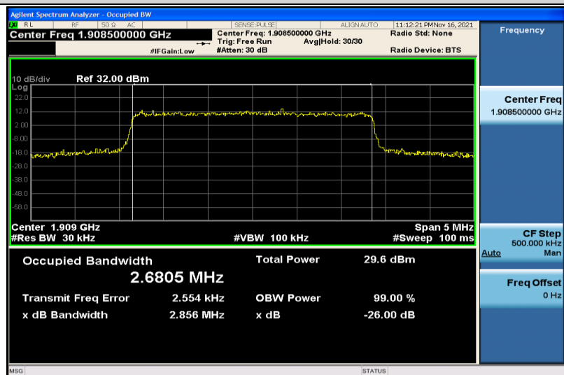
Band2-3MHz-QPSK-19185-15RB#0-2.6805
