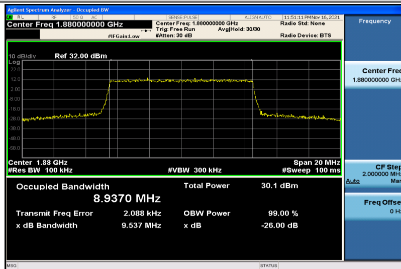
Band2-10MHz-QPSK-18900-50RB#0-8.9370
