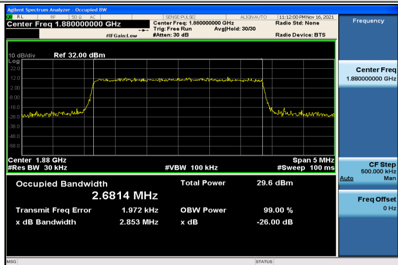
Band2-3MHz-QPSK-18900-15RB#0-2.6814
