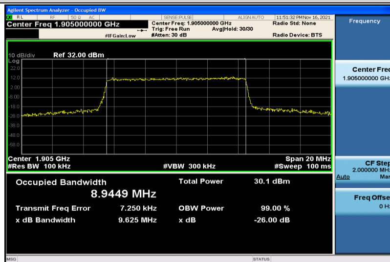
Band2-10MHz-QPSK-19150-50RB#0-8.9449
