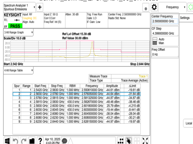
Band41_20MHz_QPSK_RB1_99_CH40620
