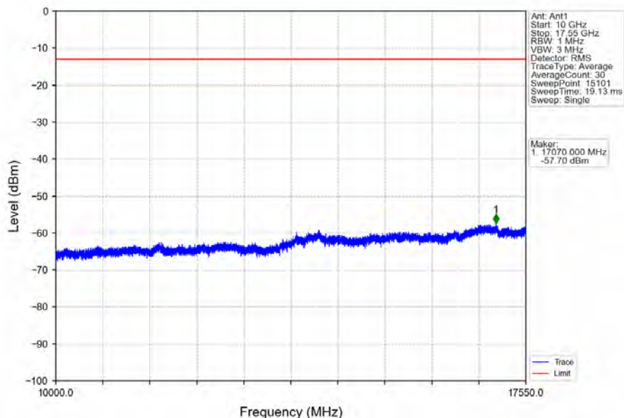
Band4_20MHz_QPSK_MCH_1732.5MHz_RB_1_0_NTNV
