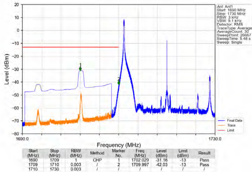
Band4_20MHz_16QAM_LCH_1720MHz_RB_1_0_NTNV
