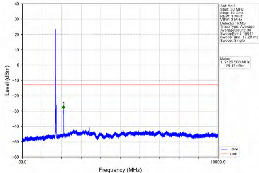
Band4_20MHz_QPSK_MCH_1732.5MHz_RB_1_0_NTNV
