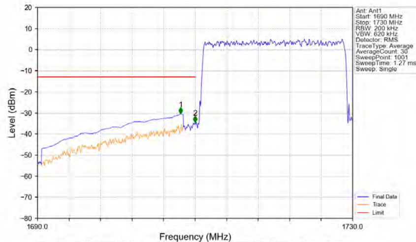
Band4_20MHz_16QAM_LCH_1720MHz_RB_100_0_NTNV
