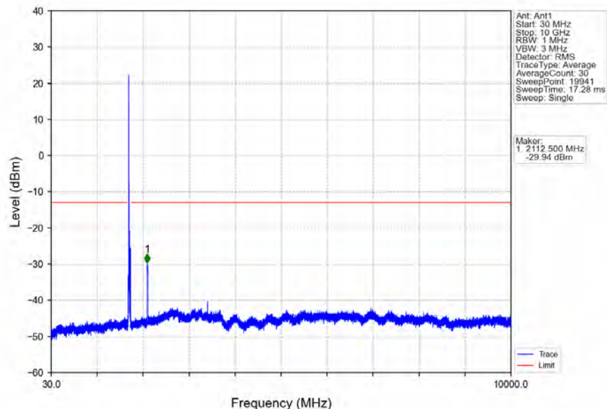
Band4_20MHz_16QAM_LCH_1720MHz_RB_1_0_NTNV
