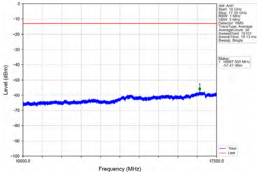
Band4_20MHz_QPSK_LCH_1720MHz_RB_100_0_NTNV
