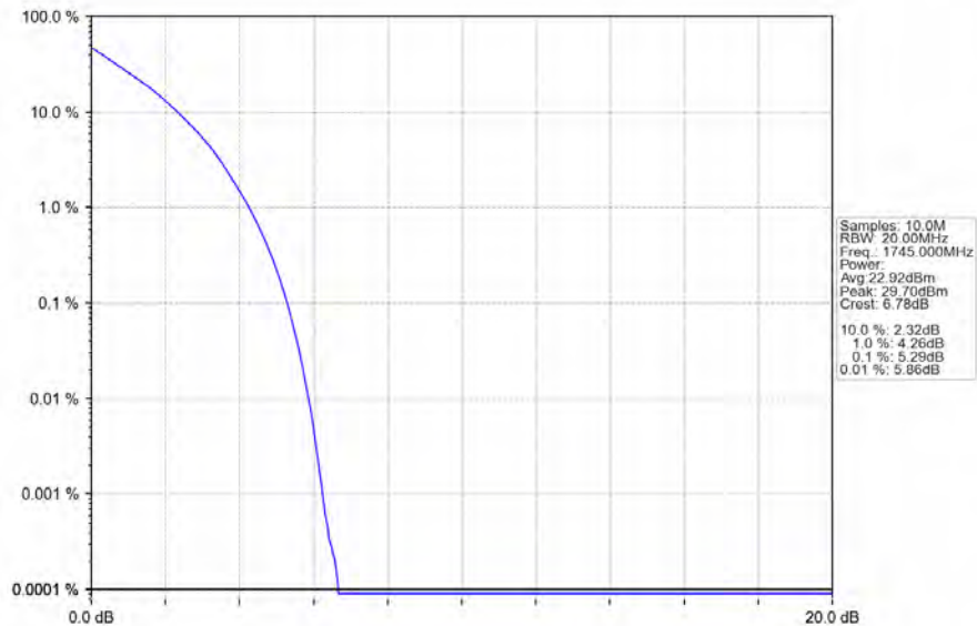
Band4_20MHz_QPSK_HCH_1745MHz_RB_100_0_NTNV
