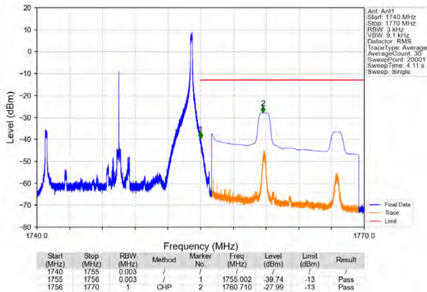
Band4_15MHz_QPSK_HCH_1747.5MHz_RB_1_74_NTNV
