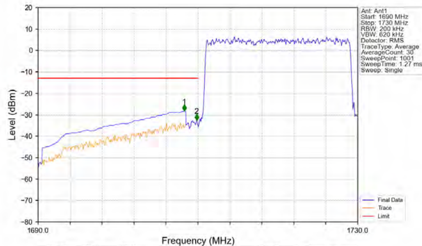
Band4_20MHz_QPSK_LCH_1720MHz_RB_100_0_NTNV
