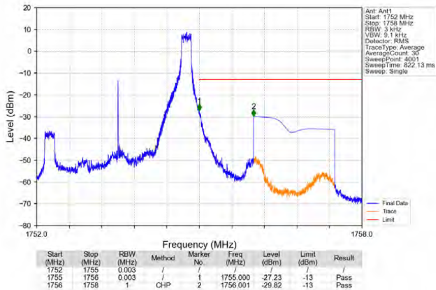
Band4_3MHz_QPSK_HCH_1753.5MHz_RB_1_14_NTNV
