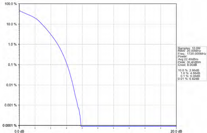
Band4_20MHz_16QAM_LCH_1720MHz_RB_100_0_NTNV
