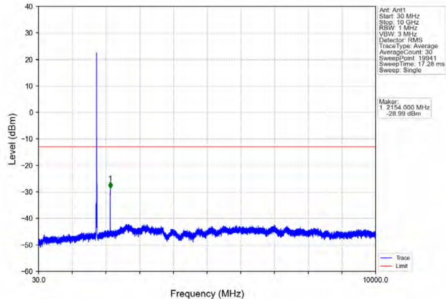
Band4_10MHz_QPSK_HCH_1750MHz_RB_1_0_NTNV
