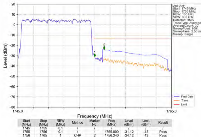
Band4_10MHz_QPSK_HCH_1750MHz_RB_50_0_NTNV
