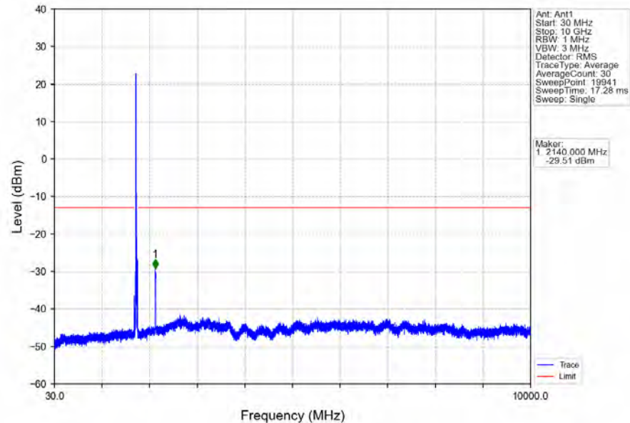
Band4_20MHz_QPSK_HCH_1745MHz_RB_1_0_NTNV
