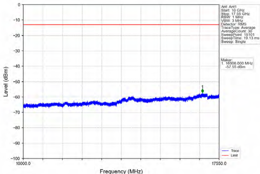
Band4_10MHz_QPSK_HCH_1750MHz_RB_1_0_NTNV
