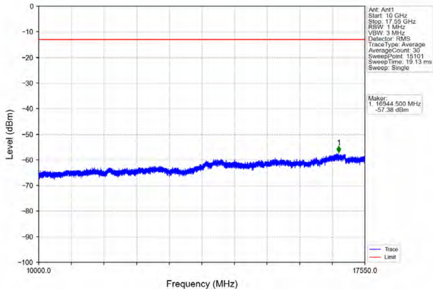
Band4_20MHz_16QAM_LCH_1720MHz_RB_100_0_NTNV
