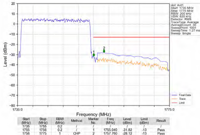
Band4_20MHz_QPSK_HCH_1745MHz_RB_100_0_NTNV
