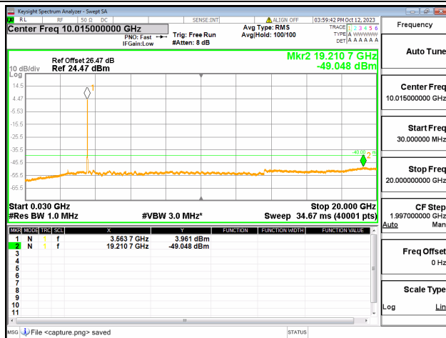
48C-30M-20G / 20+10MHz / QPSK / Low CH / 100#0-50#0
