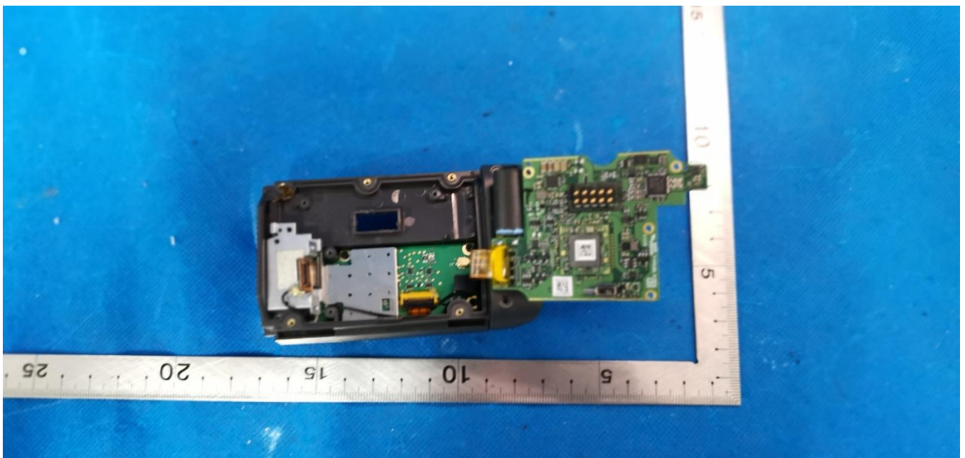
EUT Photo(12)
