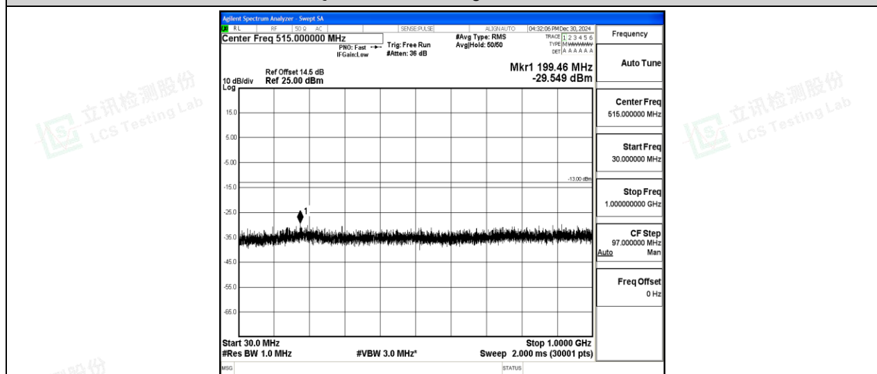
Band2-3MHz-QPSK-18615-1-0-Low-30-1000--29.55-PASS
