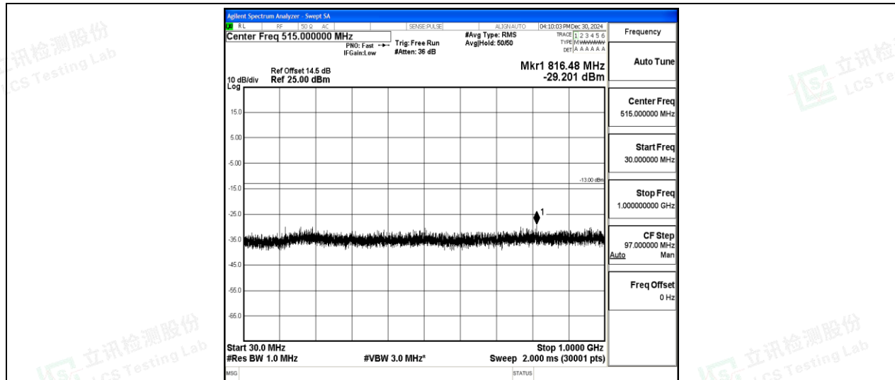
Band2-1.4MHz-16QAM-18900-1-0-Low-30-1000--29.2-PASS
