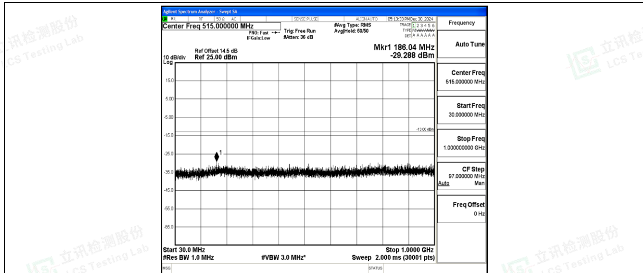
Band2-5MHz-QPSK-18900-1-0-Low-30-1000--29.29-PASS
