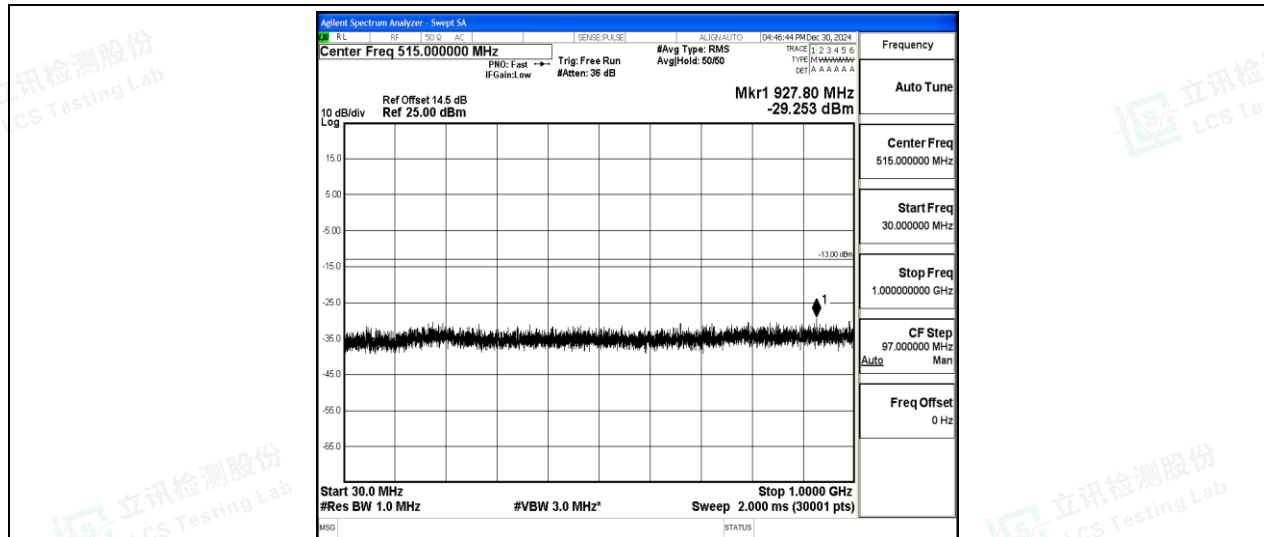
Band2-3MHz-QPSK-18900-1-0-Low-30-1000--29.25-PASS
