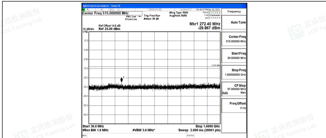
Band2-3MHz-16QAM-18900-1-0-Low-30-1000--29.87-PASS
