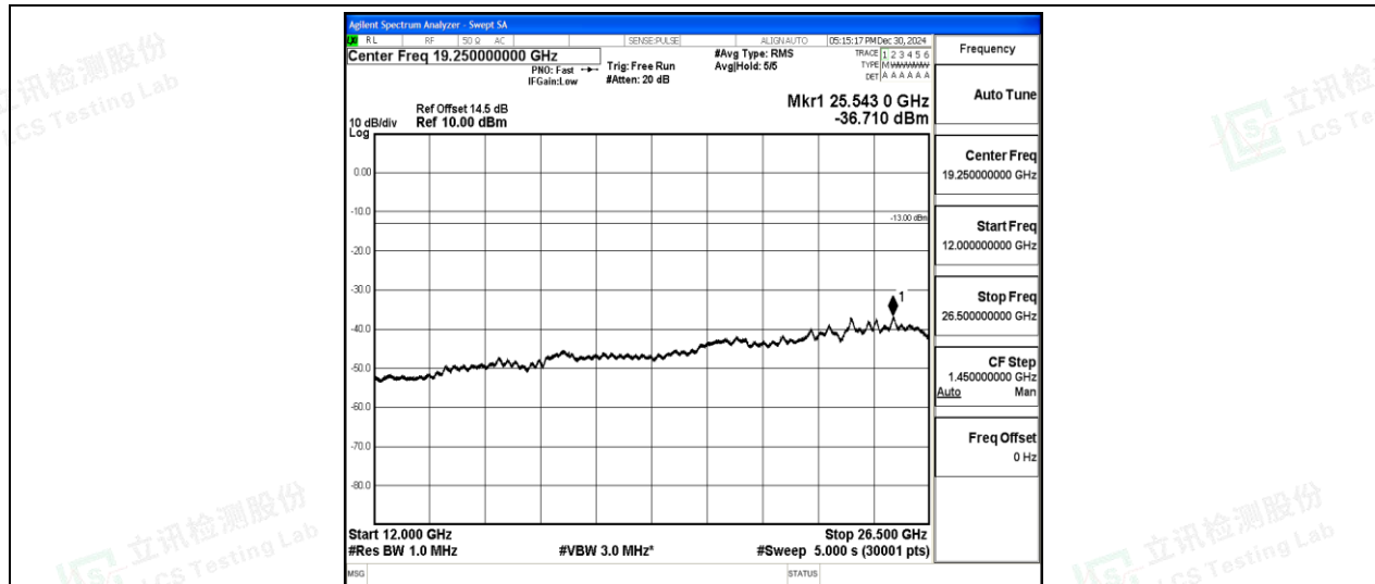
Band2-5MHz-QPSK-18900-1-0-Low-12000-26500--36.71-PASS
