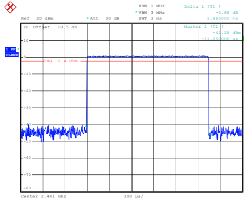
DH3_Hopping 1.665ms
