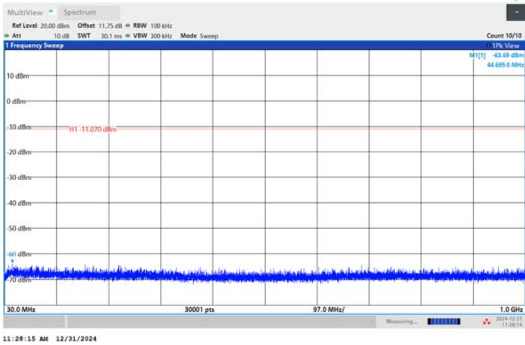
BLE_2M-Ant1-2404-30~1000-PASS
