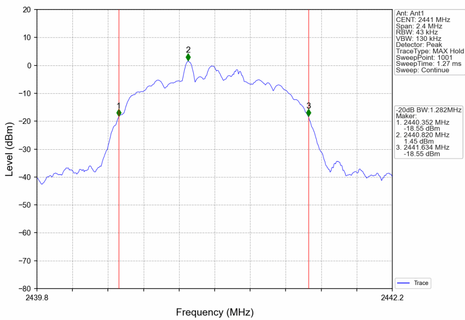
8DPSK 3DH5 MCH 2441MHz Ant1 NTV
