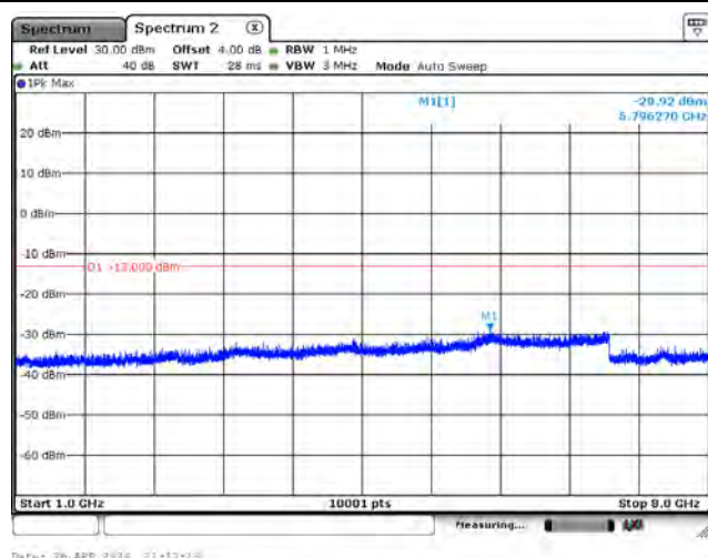
CH23278_3.75k_QPSK_1RB0_Above 1G
