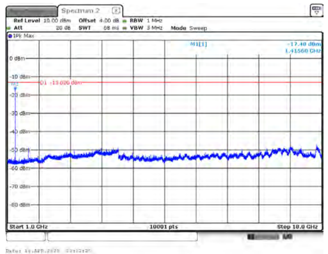
CH23278_15k_QPSK_1RB0_Above 1G
