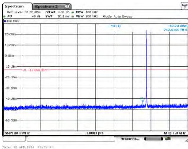
CH23278_15k_QPSK_1RB0_Below 1G
