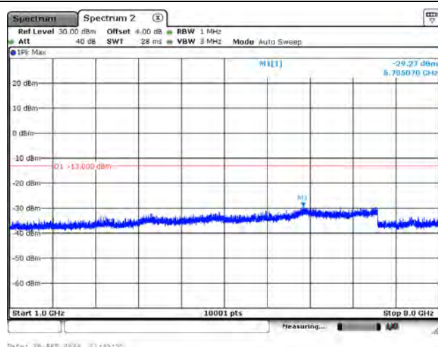
CH134180_3.75k_QPSK_1RB0_Above 1G
