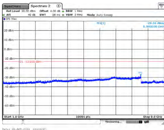
CH23178_15k_QPSK_1RB0_Above 1G
