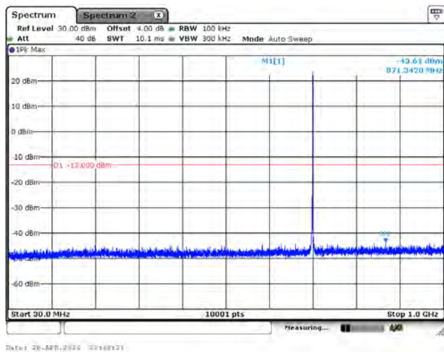
CH23178_3.75k_QPSK_1RB0_Below 1G
