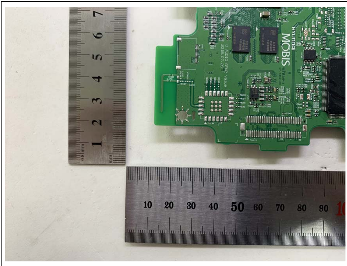
<Antenna>
