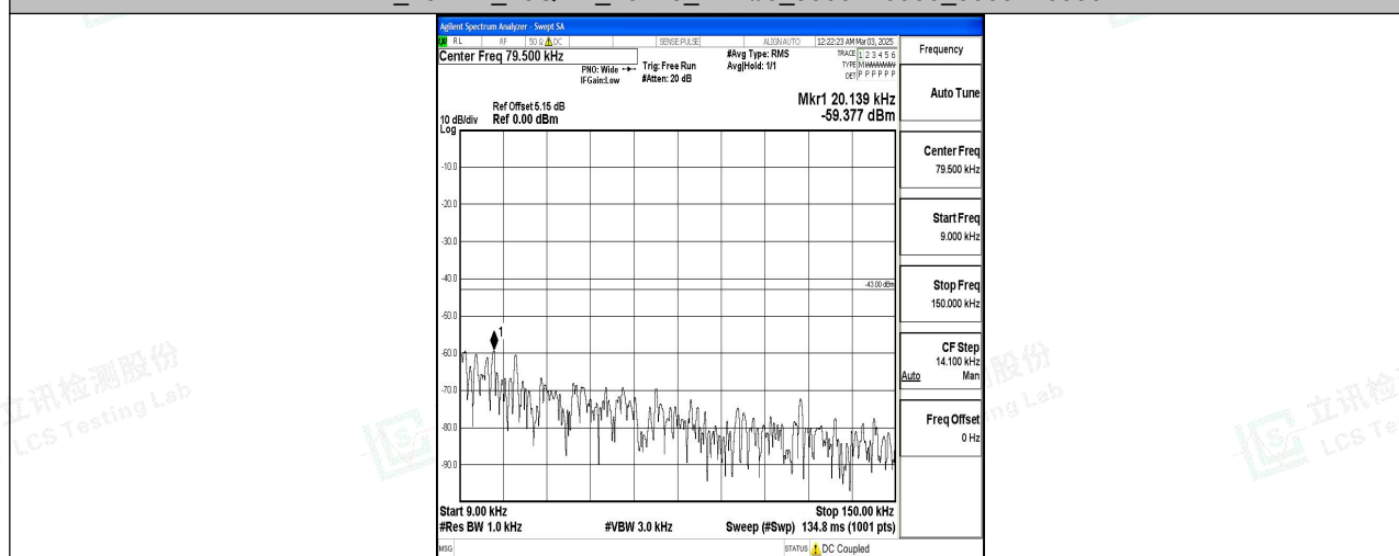
Band4 20MHz QPSK 20300 1RB#0 0.009~0.15 0.009~0.15
