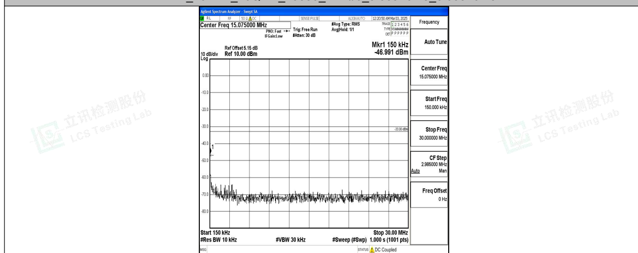
Band4 20MHz 16QAM 20050 1RB#0 0.15~30 0.15~30
