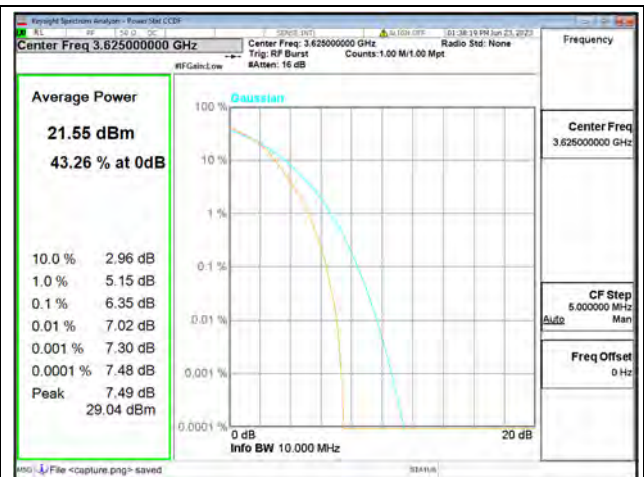
Band48 / 10MHz / Mid CH / 16QAM
