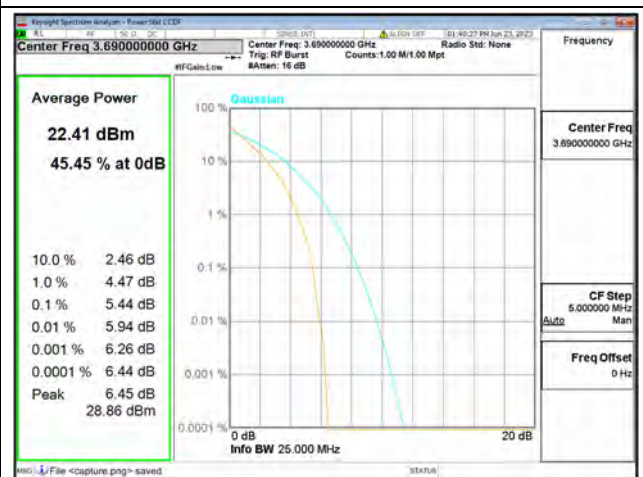
Band48 / 20MHz / High CH / QPSK
