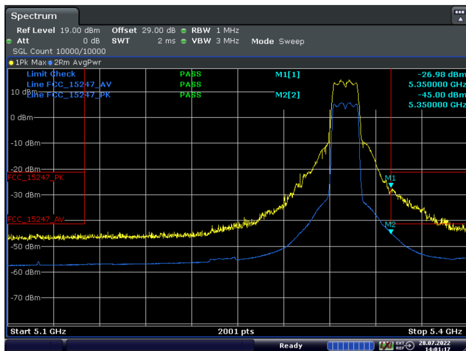
Antenna A
