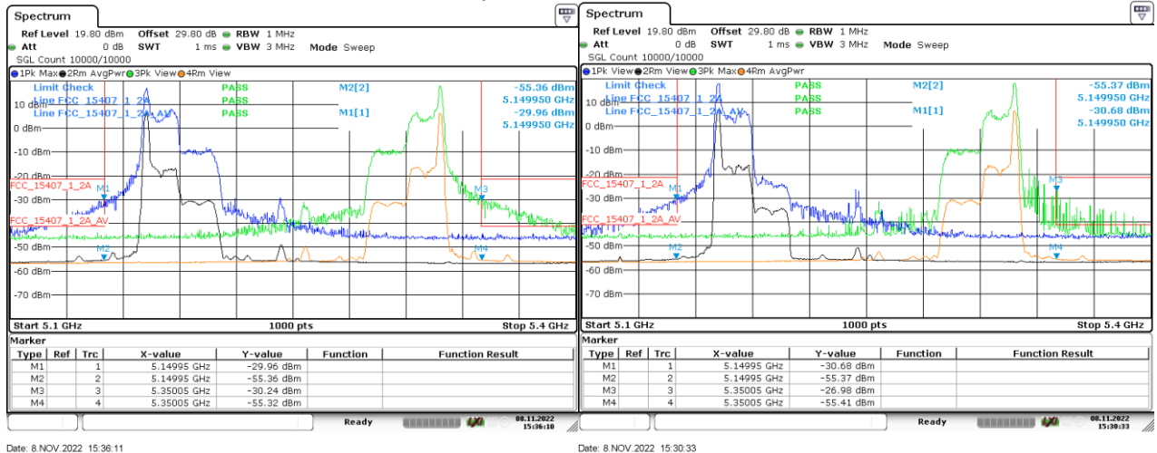
Antenna A
