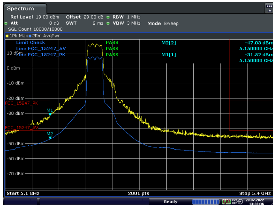
Antenna A
