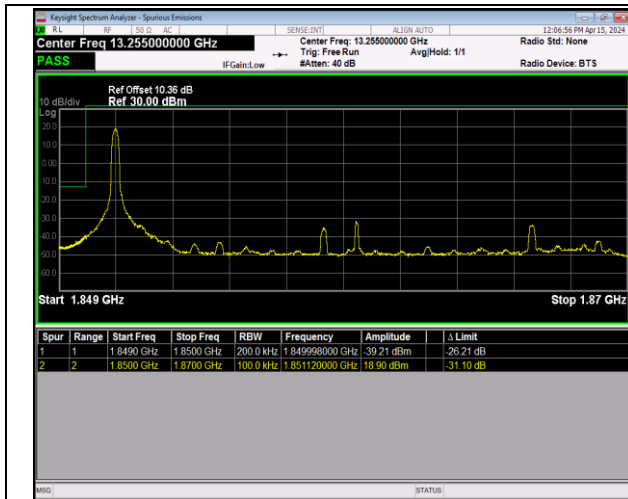
Band2_20MHz_QPSK_18700_1RB#0
