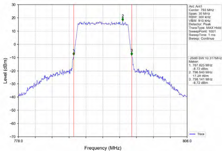
Band14_10MHz_QPSK_MCH_793MHz_RB_50_0_NTNV
