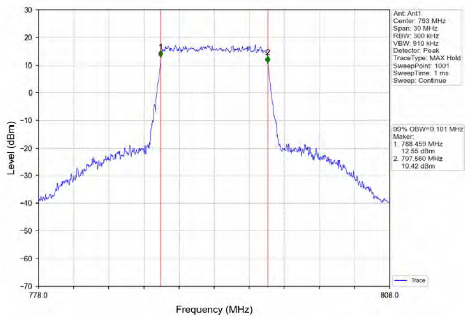
Band14_10MHz_QPSK_MCH_793MHz_RB_50_0_NTNV
