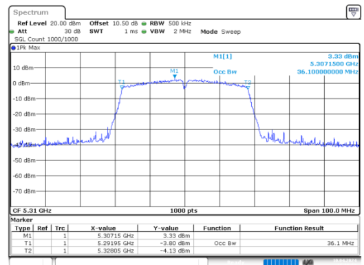
n40_5310MHz_Chain 0
