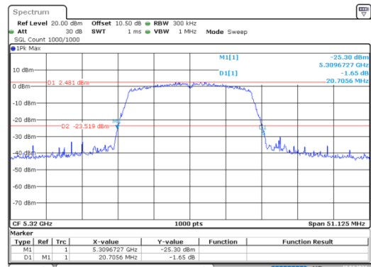
n20_5320MHz_Chain 0
