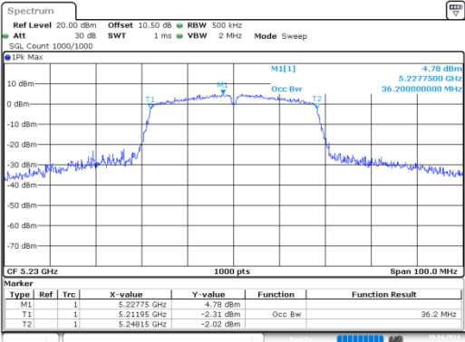
n40_5230MHz_Chain 0
