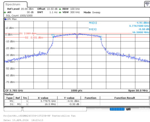
a_ 5785MHz_Chain 0
