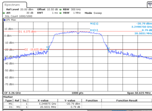
a_5260MHz_Chain 0
