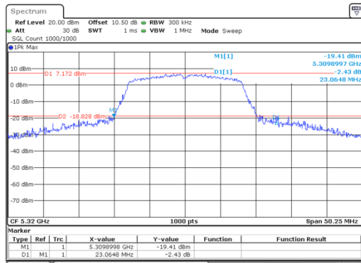
a_5320MHz_Chain 0
