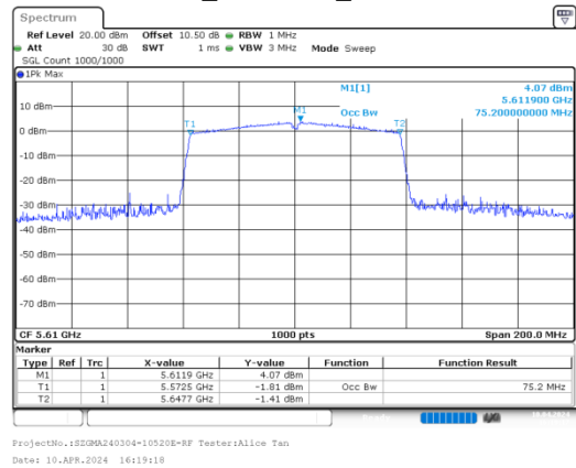
ac80_5610MHz_Chain 0
