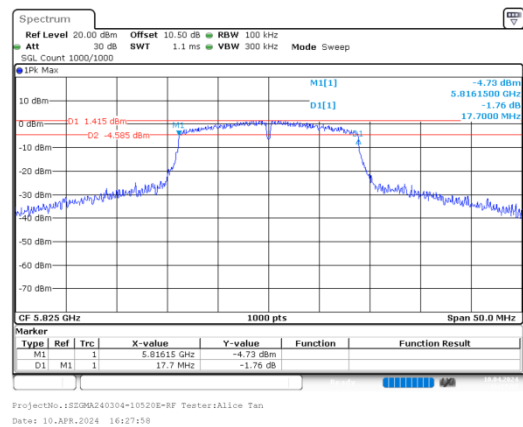
n20_ 5825MHz_Chain 0
