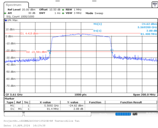
ac80_5610MHz_Chain 0
