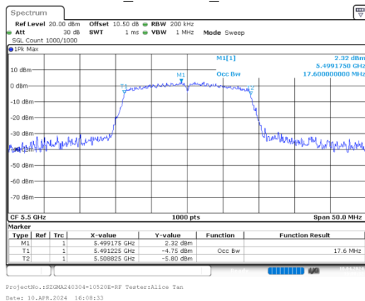
n20_5500MHz_Chain 0
