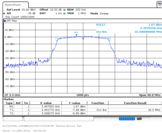
a_5500MHz_Chain 0
