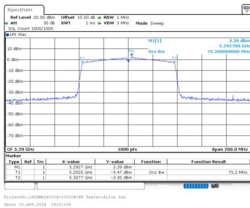
ac80_5290MHz_Chain 0
