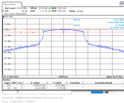
a_ 5825MHz_Chain 0
