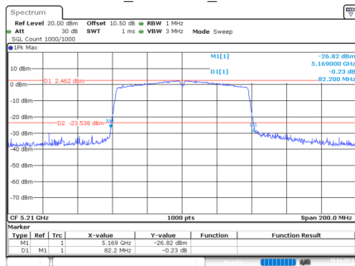
ac80_5210MHz_Chain 0
