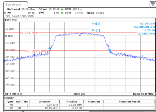
a_5280MHz_Chain 0
