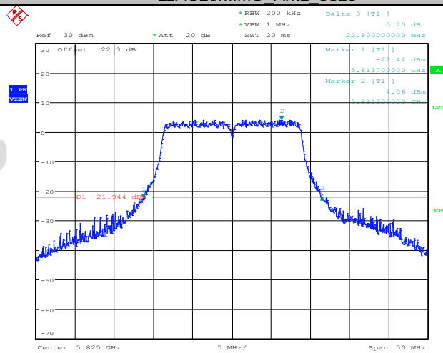
11AC20MIMO_Ant1_5825
