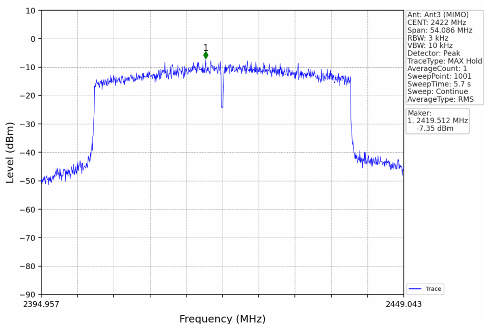
802.11ax(HEW40)_LCH_2422MHz_RU484_Left_Ant3 (MIMO)_NTNV
