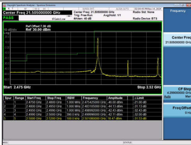
Band7_20MHz_QPSK_20850_1RB#0
