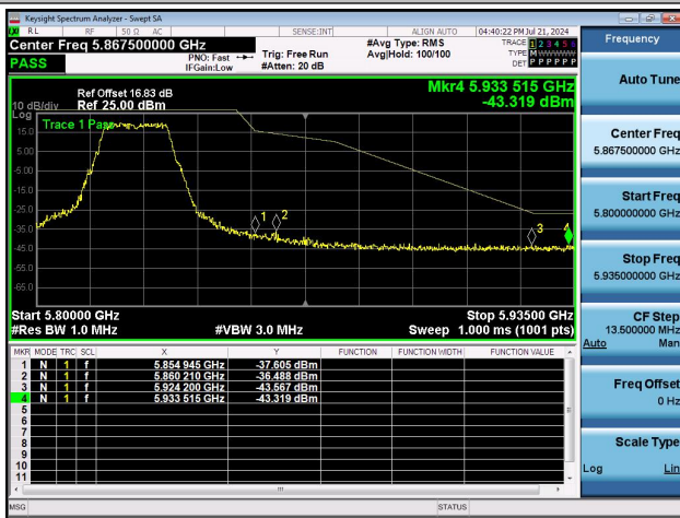
11A-Ant0-5825-PASS
