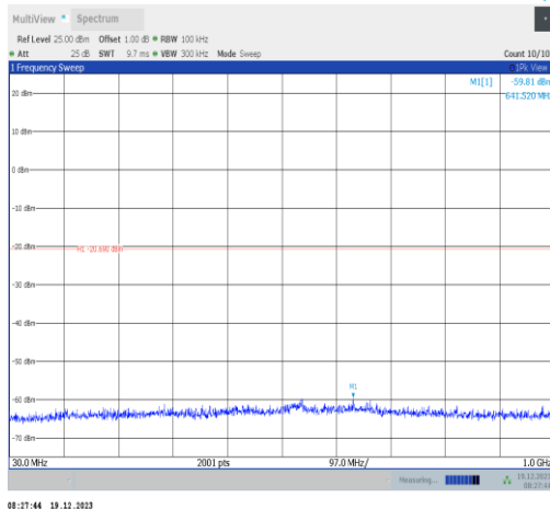
11ax20MIMO-Ant3-2437-30~1000-PASS
