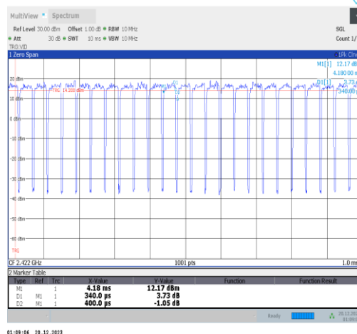
NTNV-11ax40MIMO-Ant3-2422
