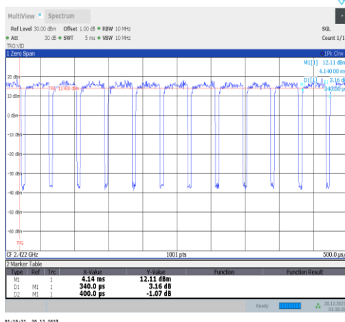
NTNV-11ax40MIMO-Ant4-2422
