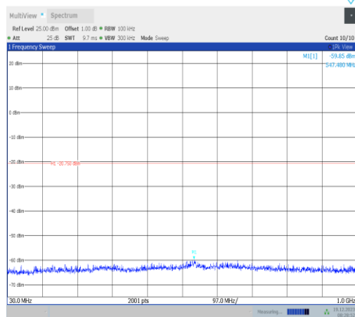
11ax20MIMO-Ant4-2437-30~1000-PASS
