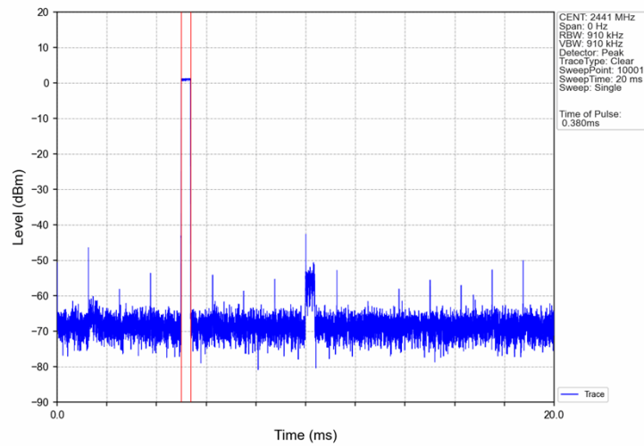
GFSK_DH1_HOPP_Ant1_NTNV
