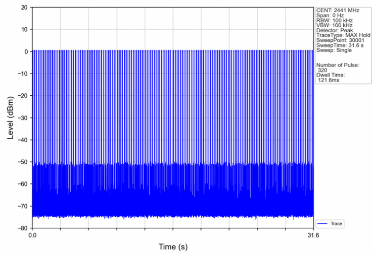
GFSK_DH1_HOPP_Ant1_NTNV
