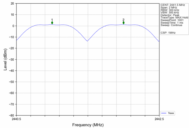
Pi/4DQPSK_2DH5_HOPP_Ant1_NTV
