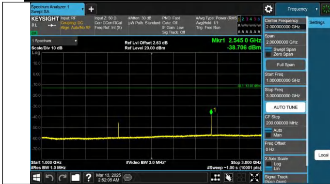
Band26(824-849)-10MHz-QPSK-26990-1RB#49-1000~3000-PAS
