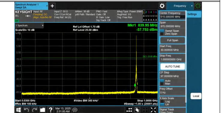
Band26(824-849)-3MHz-QPSK-27025-1RB#14-30~1000-PASS
