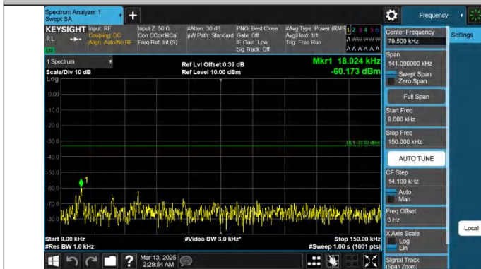
Band26(824-849)-3MHz-QPSK-27025-1RB#0-0.009~0.15-PASS
