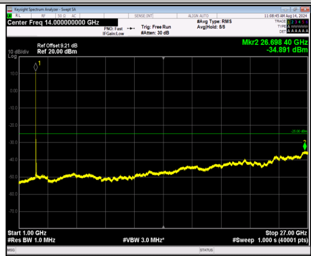
7-7-20MHz-20MHz-QPSK-QPSK-21001-21199-1RB#0-1RB #99-1000~27000MHz-PASS
