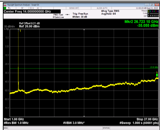
7-7-20MHz-20MHz-QPSK-QPSK-20850-21048-1RB#99-0R B#0-1000~27000MHz-PASS
