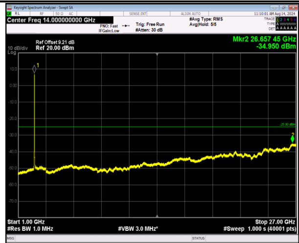
7-7-20MHz-20MHz-QPSK-QPSK-21001-21199-100RB#0-1 00RB#0-1000~27000MHz-PASS
