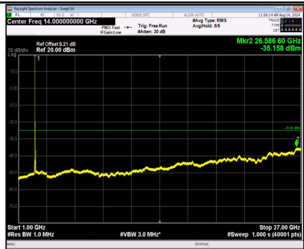
7-7-20MHz-20MHz-QPSK-QPSK-21001-21199-1RB#0-0RB #0-1000~27000MHz-PASS
