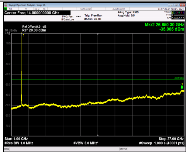
7-7-20MHz-20MHz-QPSK-QPSK-21001-21199-1RB#99-0R B#0-1000~27000MHz-PASS
