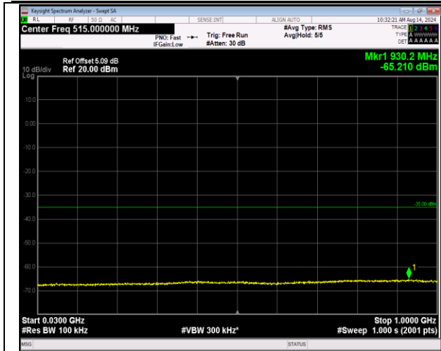
7-7-20MHz-10MHz-QPSK-QPSK-21051-21195-100RB#0 -50RB#0-30~1000MHz-PASS
