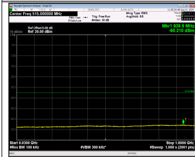
7-7-20MHz-20MHz-QPSK-QPSK-21001-21199-1RB#0-1 RB#99-30~1000MHz-PASS
