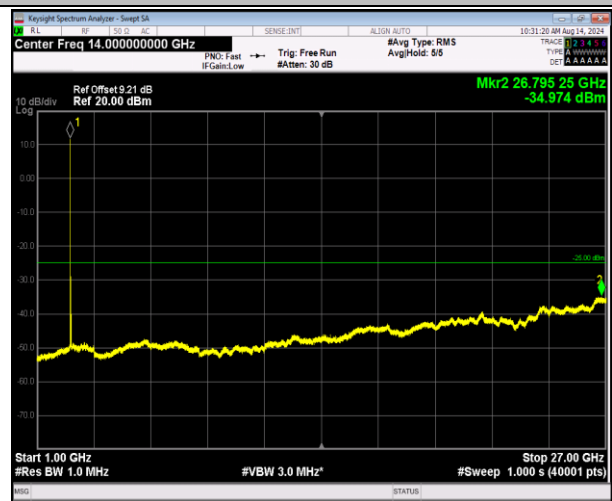
7-7-20MHz-10MHz-QPSK-QPSK-21051-21195-1RB#0-1RB #49-1000~27000MHz-PASS
