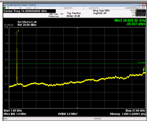
7-7-20MHz-20MHz-QPSK-QPSK-20850-21048-1RB#0-1RB #99-1000~27000MHz-PASS
