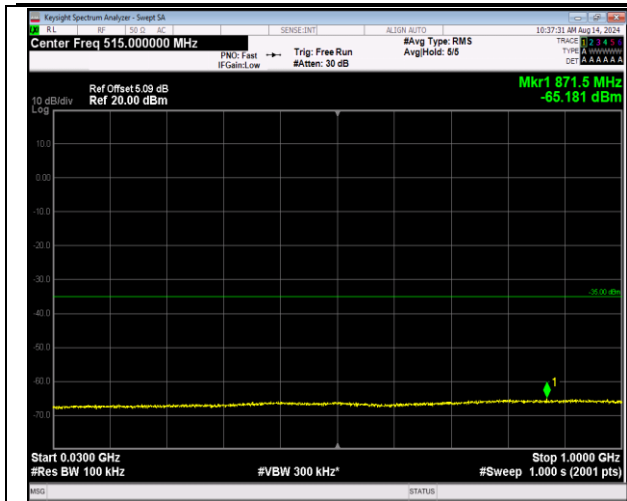
7-7-20MHz-10MHz-QPSK-QPSK-21251-21395-100RB#0 -50RB#0-30~1000MHz-PASS
