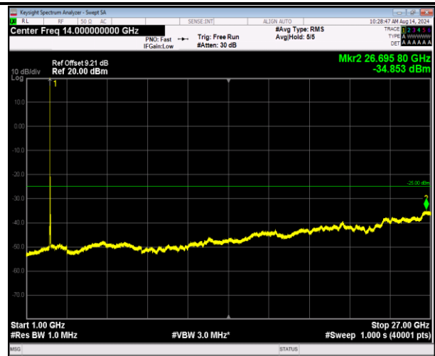
7-7-20MHz-10MHz-QPSK-QPSK-21051-21195-1RB#0-0RB #0-1000~27000MHz-PASS
