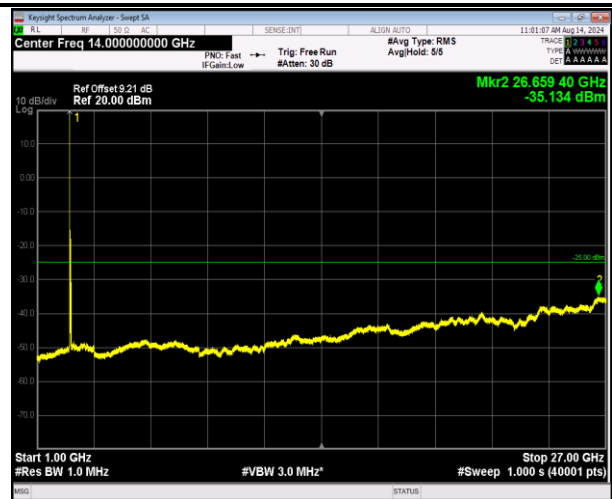
7-7-20MHz-20MHz-QPSK-QPSK-20850-21048-1RB#0-0RB #0-1000~27000MHz-PASS
