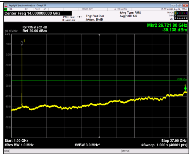
7-7-20MHz-10MHz-QPSK-QPSK-21251-21395-100RB#0-5 ORB#0-1000~27000MHz-PASS
