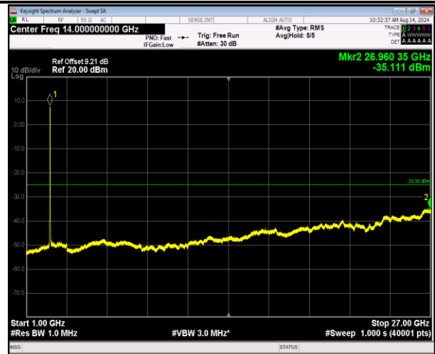
7-7-20MHz-10MHz-QPSK-QPSK-21051-21195-100RB#0-5 ORB#0-1000~27000MHz-PASS
