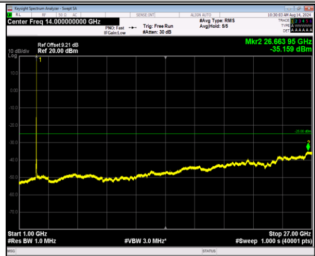
7-7-20MHz-10MHz-QPSK-QPSK-21051-21195-1RB#99-0R B#0-1000~27000MHz-PASS
