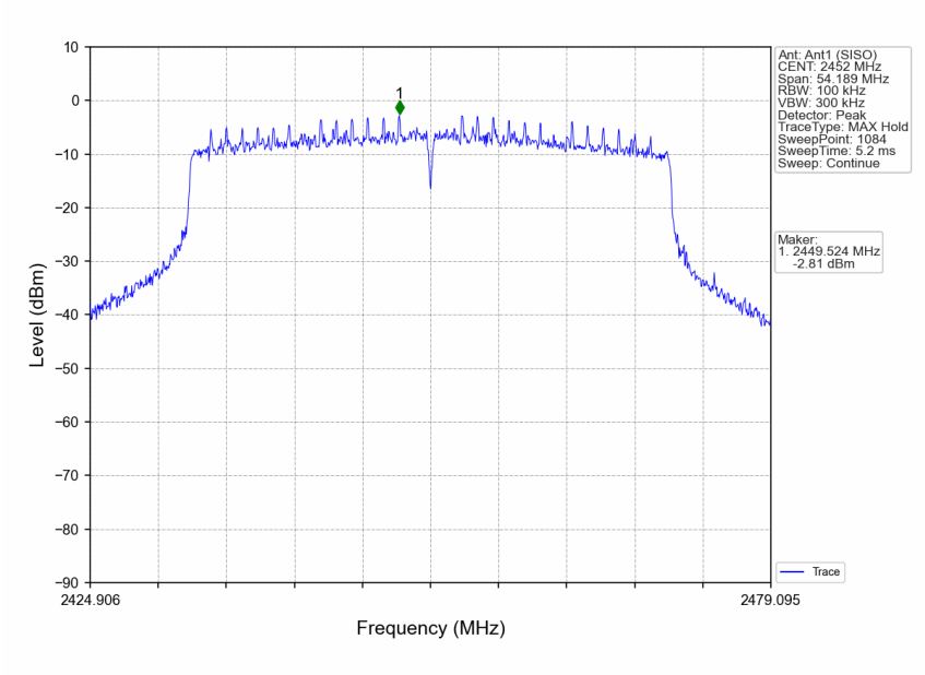
802.11ax(HEW40)_HCH_2452MHz_RU484_Left_Ant1 (SISO)_NTNV
