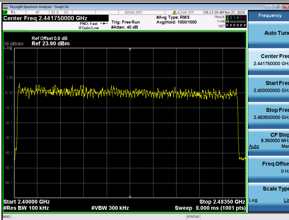
3DH5_Ant1_Hop
