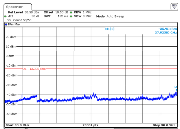
n78_3_30MHz_30kHz_3785MHz_DFT-s-OFDM QPSK_RB75@0 -35.95dBm
