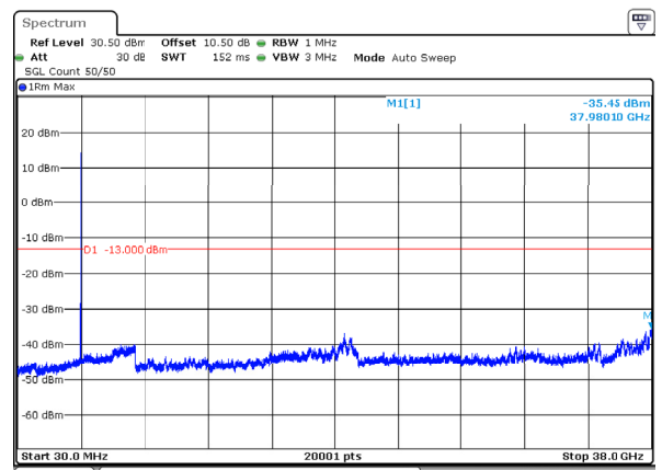
n78_3_40MHz_30kHz_3750MHz_DFT-s-OFDM QPSK_RB1@105 -35.45dBm
