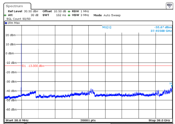
n78_3_50MHz_30kHz_3725MHz_DFT-s-OFDM QPSK_RB1@132 -35.67dBm
