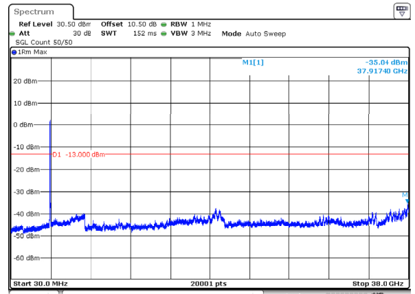
n78_3_50MHz_30kHz_3725MHz_DFT-s-OFDM QPSK_RB128@0 -35.04dBm
