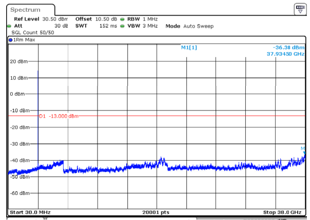
n78_3_30MHz_30kHz_3785MHz_DFT-s-OFDM QPSK_RB1@0 -36.38dBm
