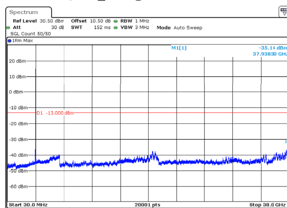
n78_3_70MHz_30kHz_3765MHz_DFT-s-OFDM QPSK_RB1@188 -35.14dBm
