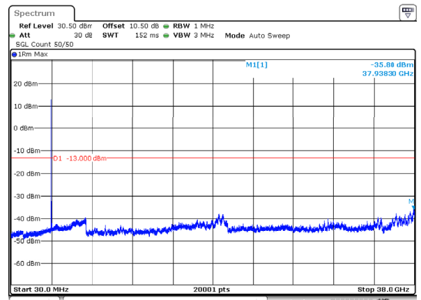
n78_3_90MHz_30kHz_3755MHz_DFT-s-OFDM QPSK_RB1@0 -35.80dBm
