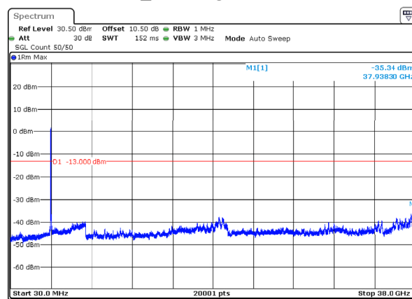
n78_3_70MHz_30kHz_3765MHz_DFT-s-OFDM QPSK_RB180@0 -35.34dBm
