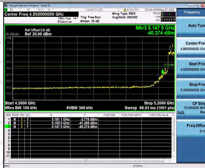
11N40ISO_Ant2_Low_5190
