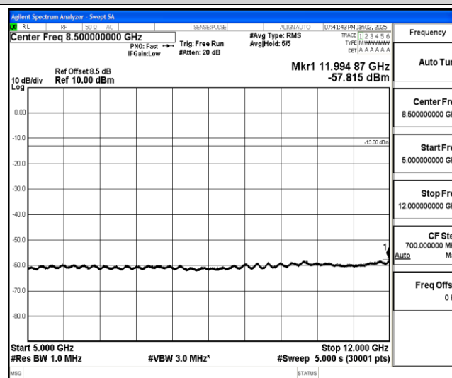
Band25-3MHz-QPSK-26365-1-0-Low-5000-12000--57.82-PASS
