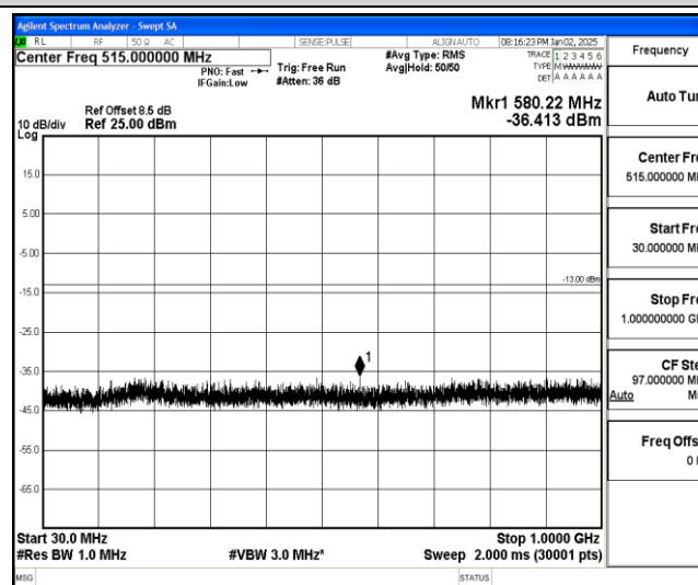
Band25-5MHz-16QAM-26065-1-0-Low-30-1000--36.41-PASS
