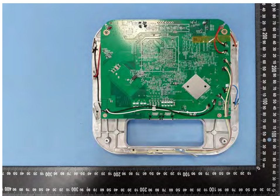
EUT Photo (12)
