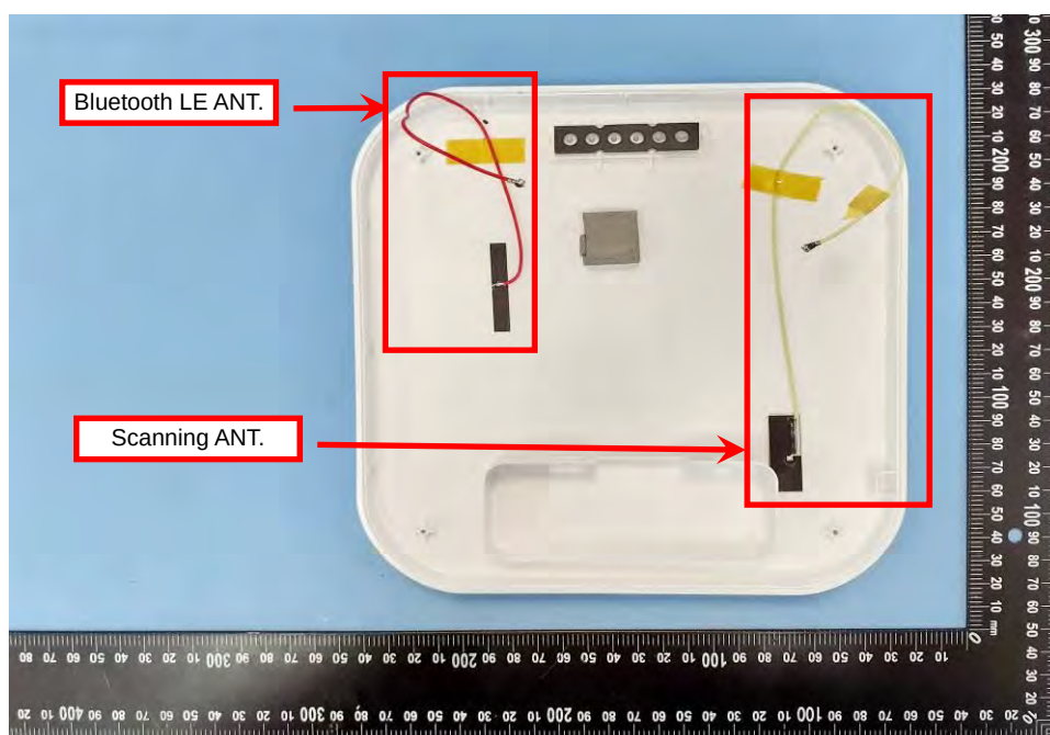
EUT Photo (2)
