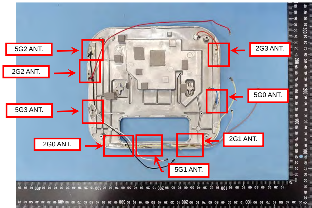
EUT Photo (18)
